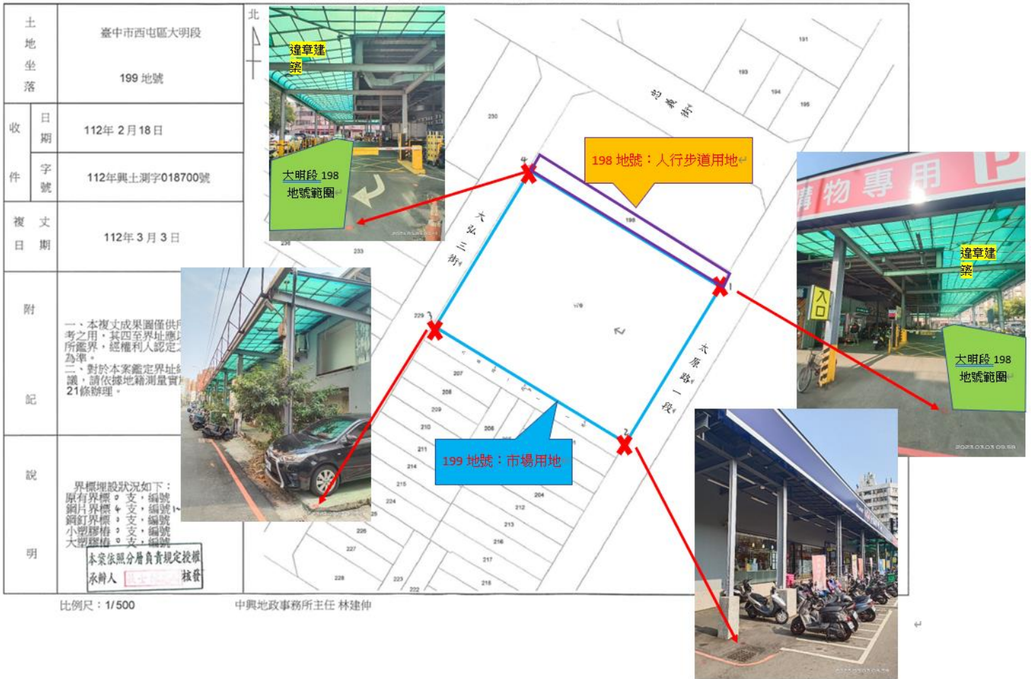
臺中市中興地政事務所 土地複丈成果圖
