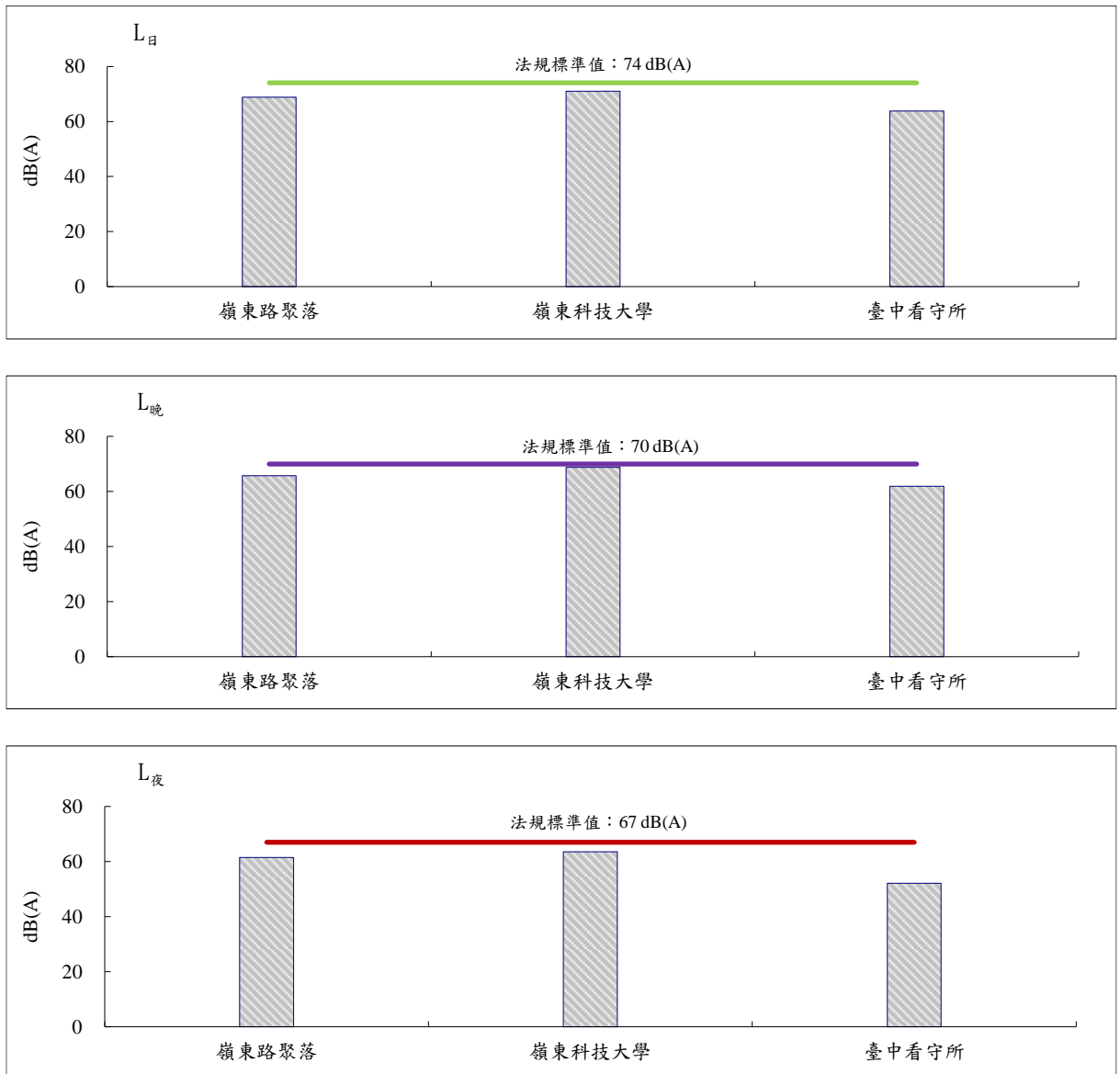
圖 2.2.1-1 本季噪音監測結果
