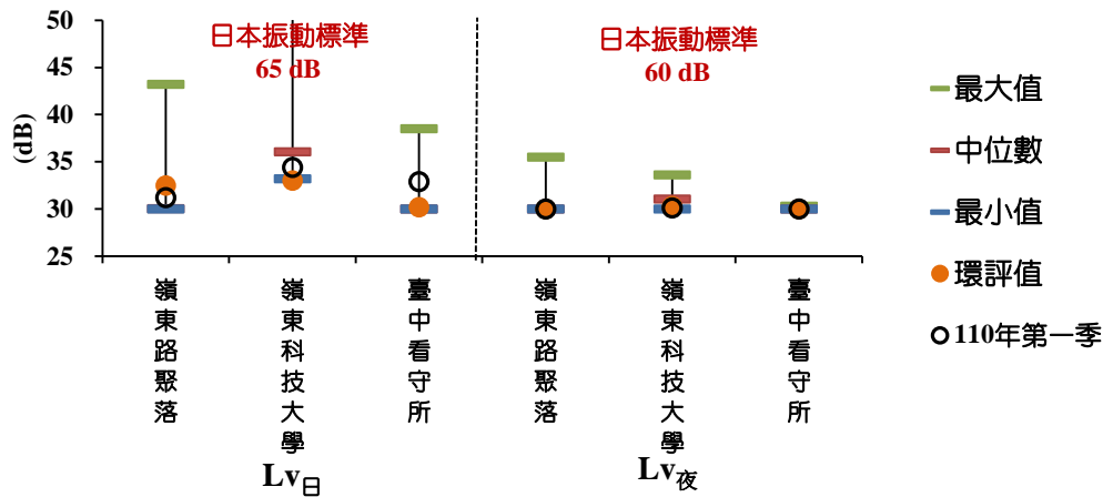
圖 2.3.2-1 歷次振動監測結果
