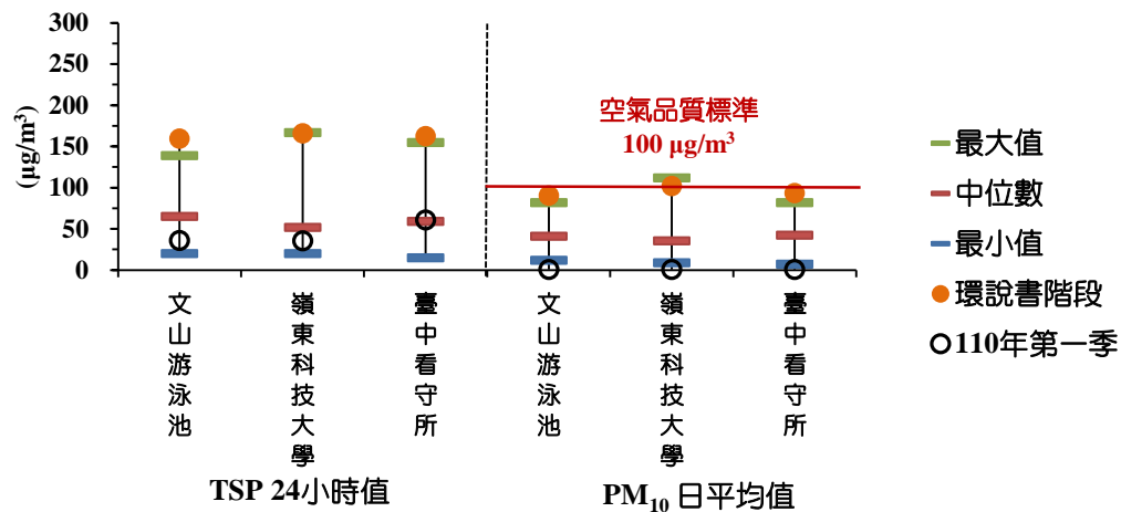
圖 2.1.2-1 歷次空氣品質監測結果(續 1)
