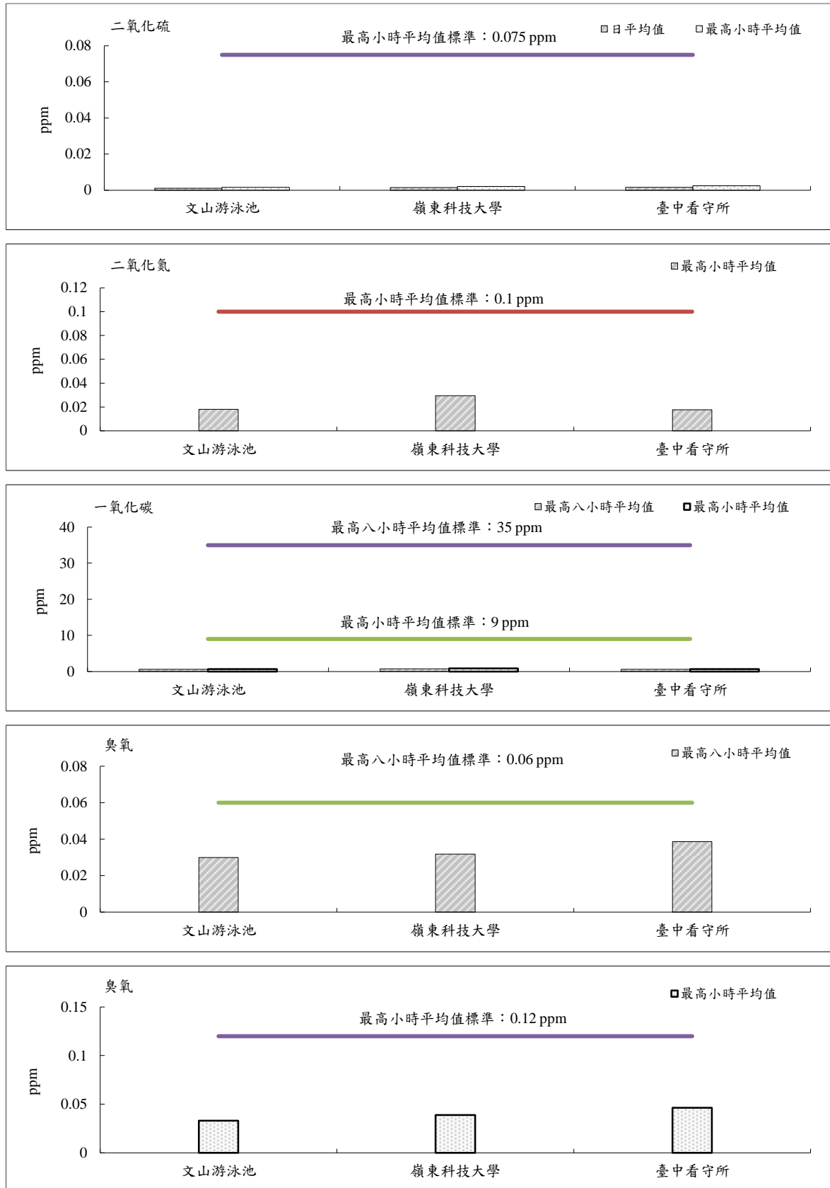
圖 2.1.1-1 本季空氣品質監測結果
