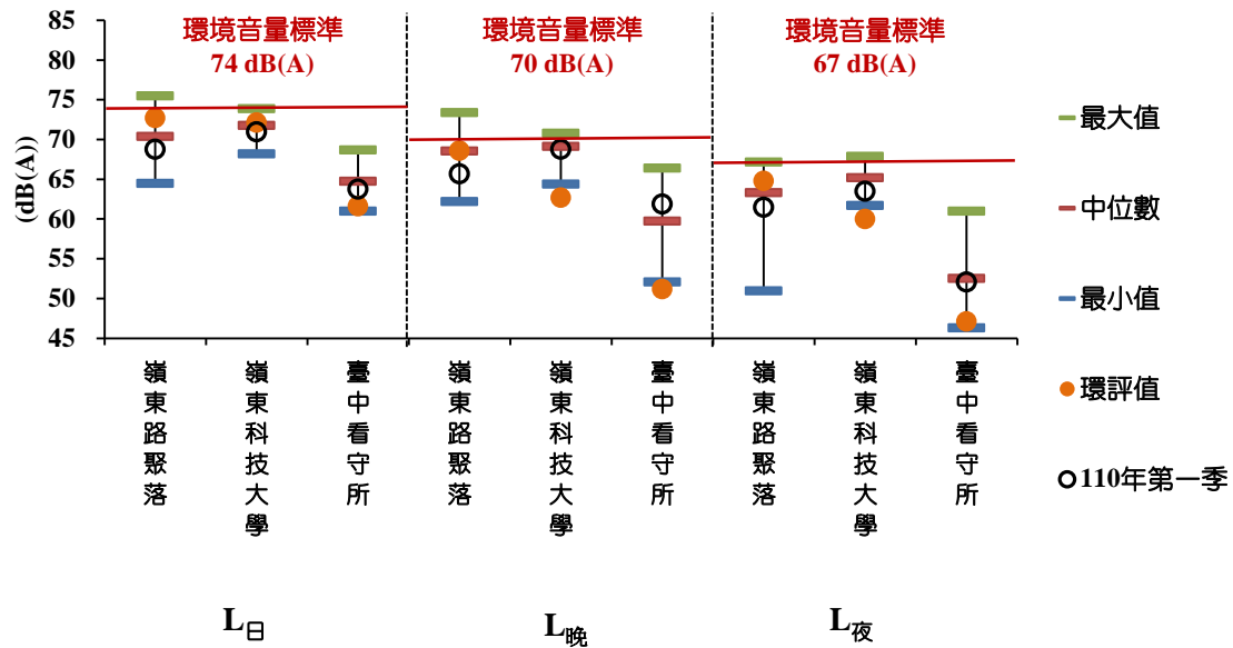
圖 2.2.2-1 歷次噪音監測結果
