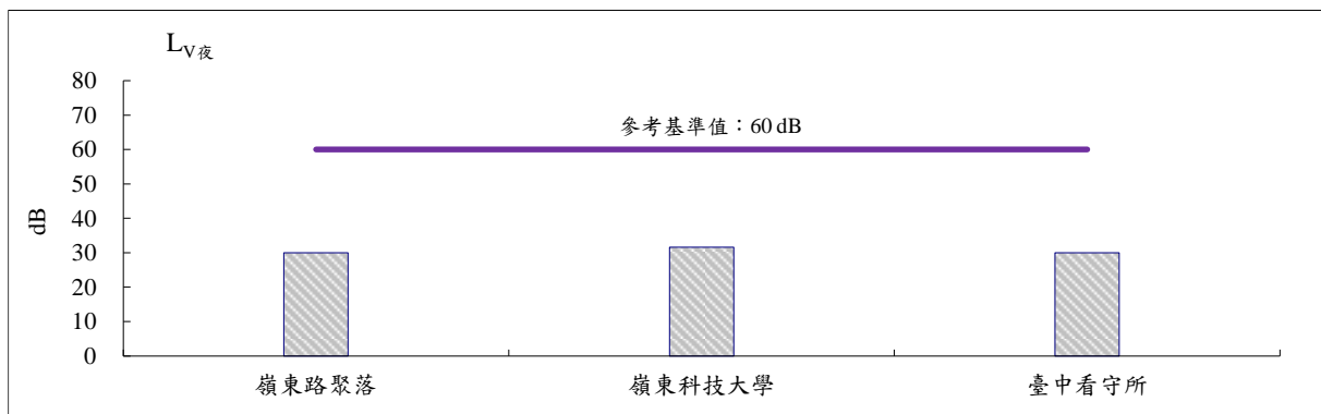
圖 2.3.1-1 本季振動監測結果
