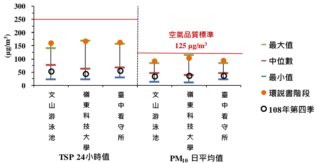
圖 2.1.2-1 歷次空氣品質監測結果(續 1)
