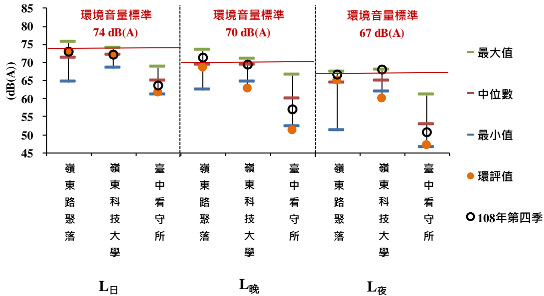
圖 2.2.2-1 歷次噪音監測結果
