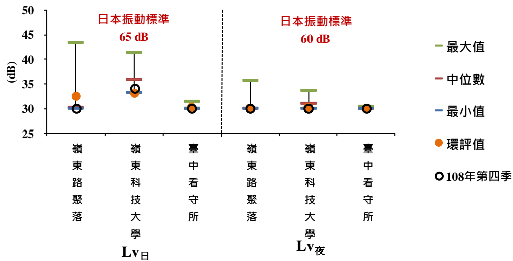
圖 2.3.2-1 歷次振動監測結果
