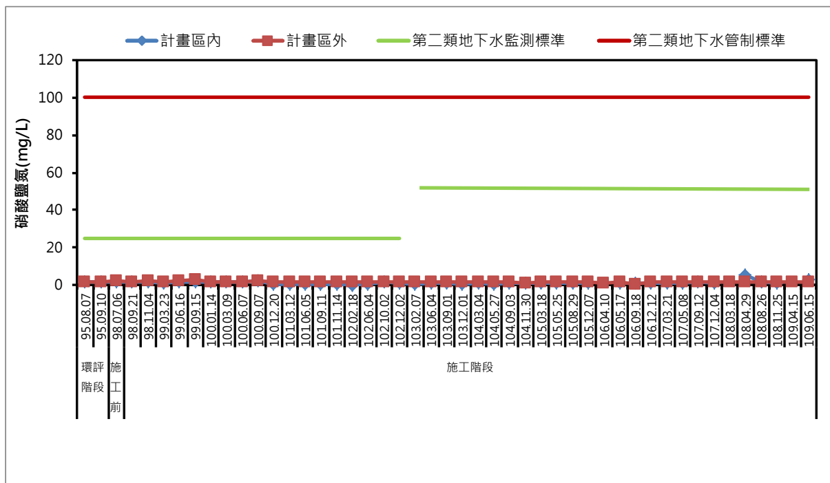
圖 3.1.1-30、歷次地下水質硝酸鹽氮監測結果
