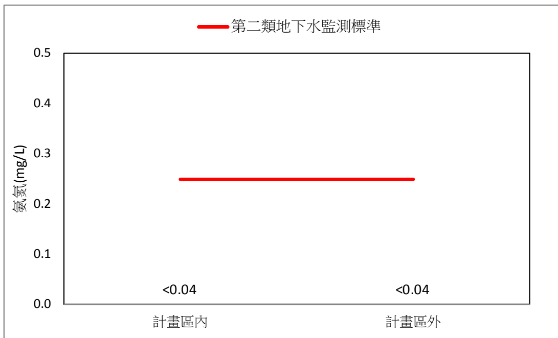
圖 2.2-4、109 年第二季地下水質氨氮監測比較圖
