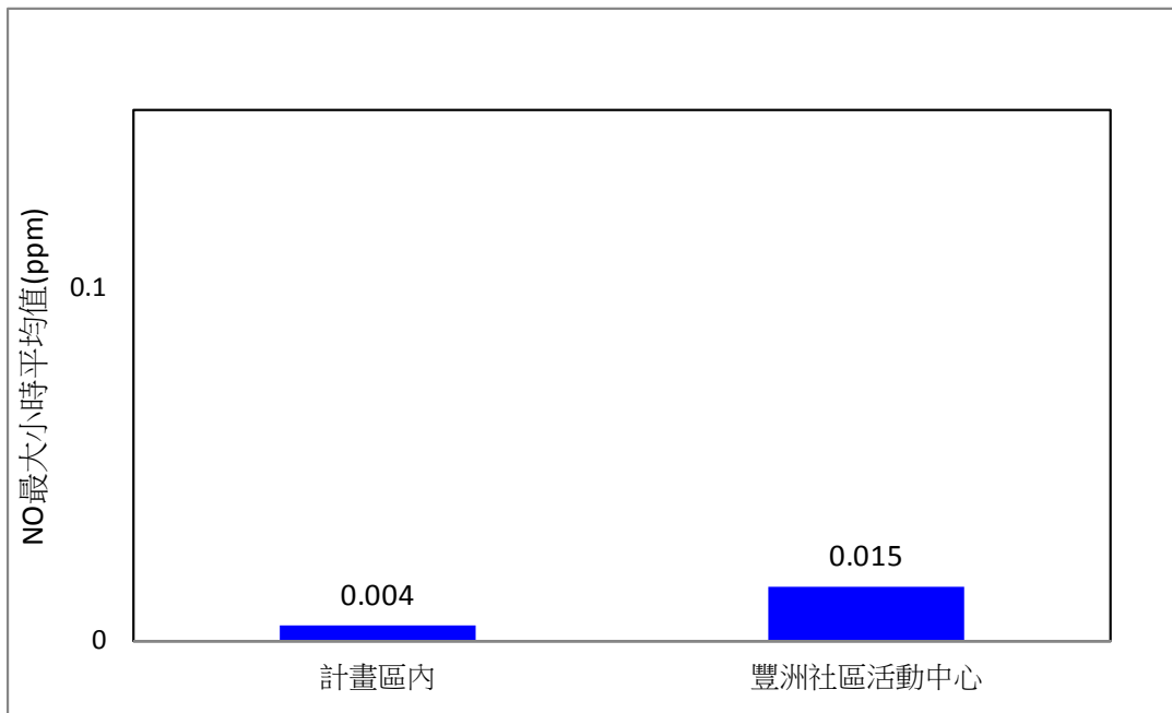
圖 2.3-7、109 年第二季空氣品質 NO 最大小時平均值監測比較圖
