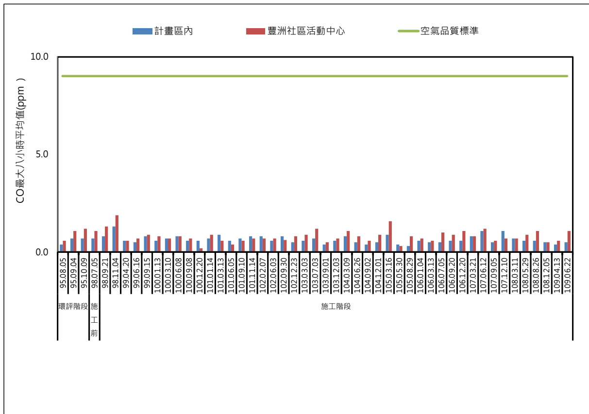
圖 3.1.1-51、歷次空氣品質 CO 最大八小時平均值監測結果
