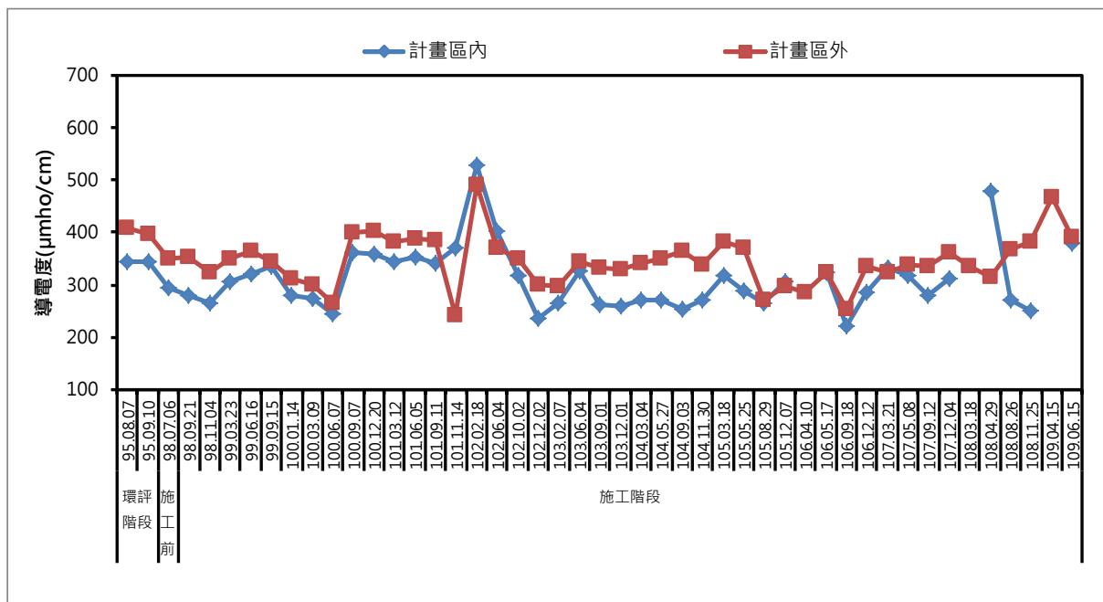
圖 3.1.1-28、歷次地下水質導電度監測結果
