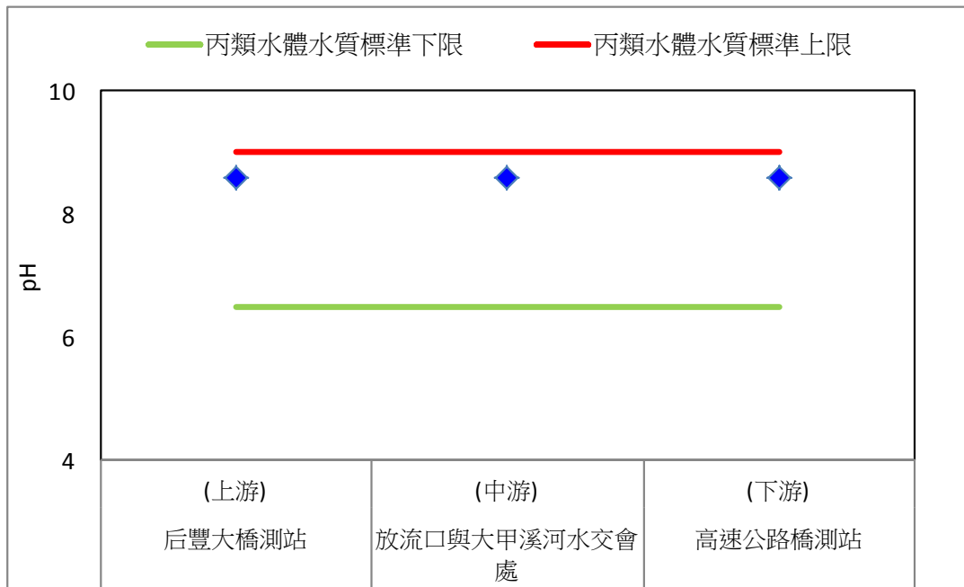
圖 2.1-1、109 年第二季地面水質 pH 值監測比較圖
