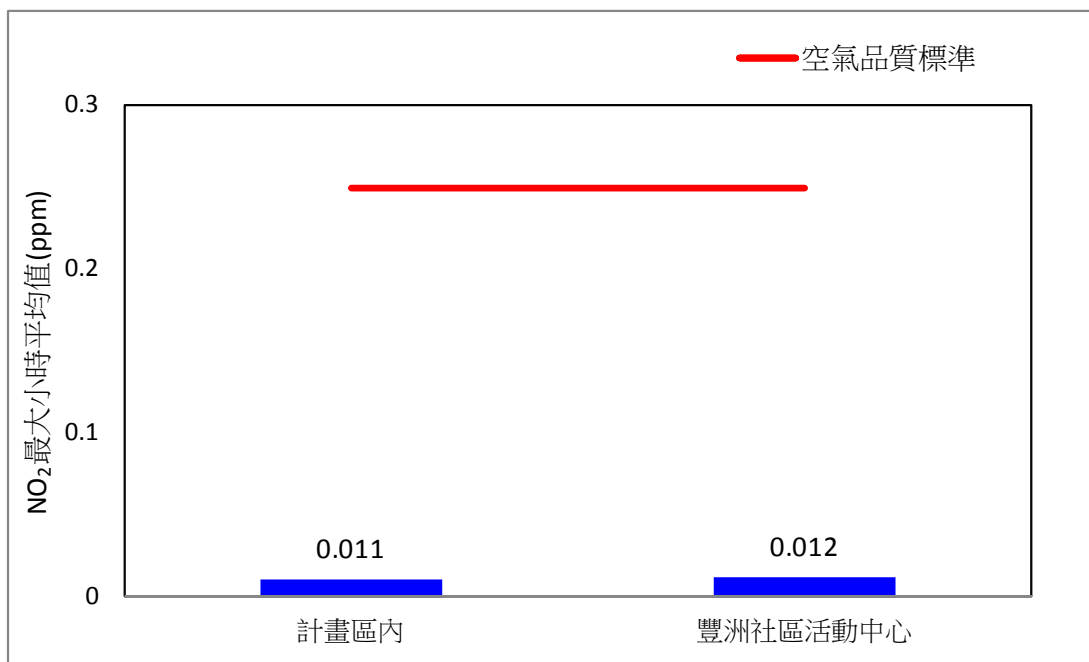
圖 2.3-8、109 年第二季空氣品質 NO 2 最大小時平均值監測比較圖
