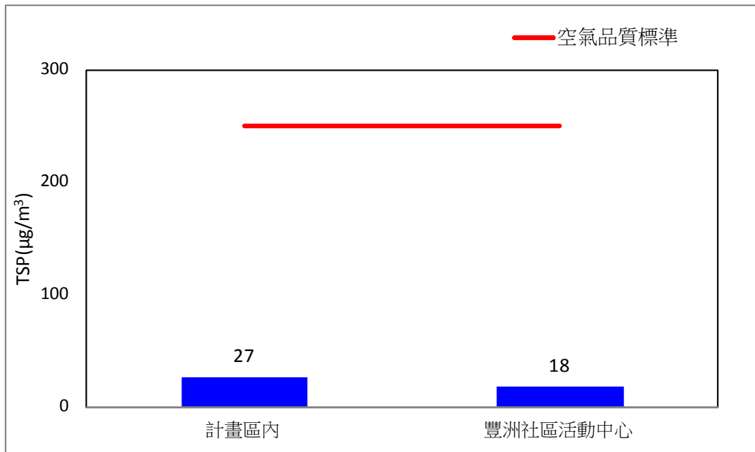
圖 2.3-1、109 年第二季空氣品質 TSP 監測比較圖
