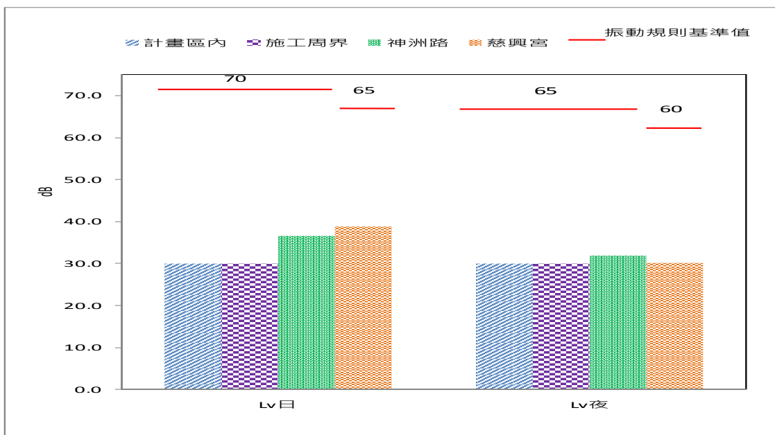
圖 2.5-2、109 年第二季各時段振動監測值比較圖
