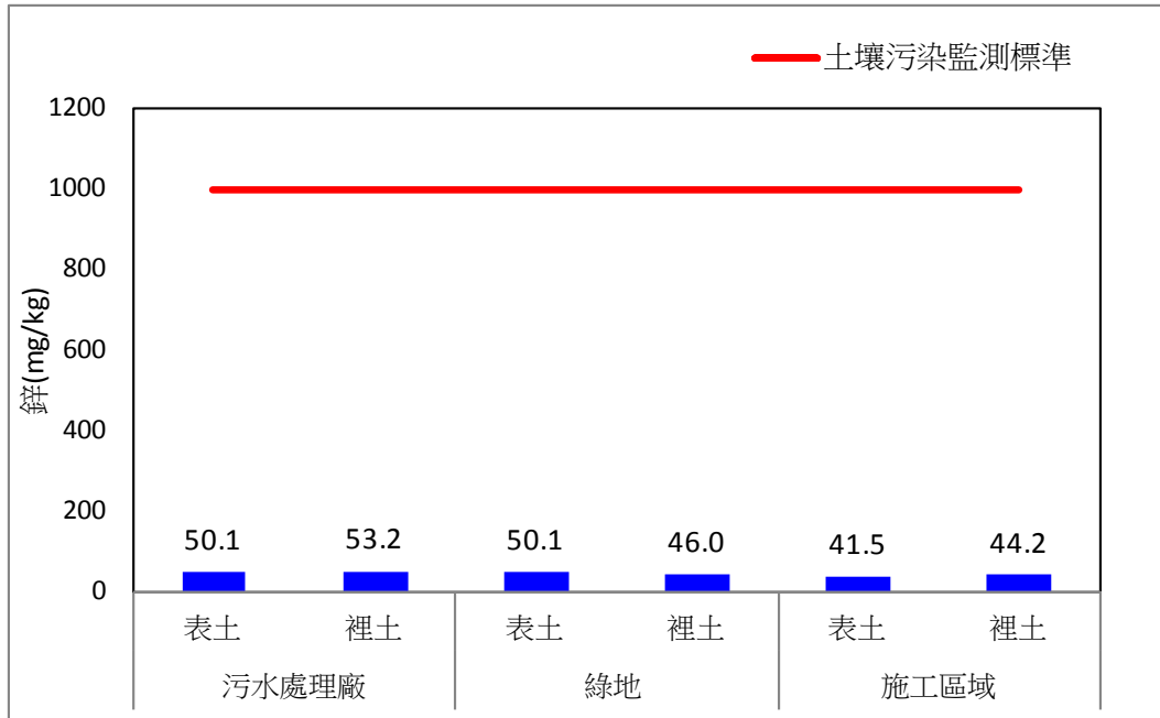
圖 2.4-3、109 年第二季土壤重金屬鋅監測比較圖
