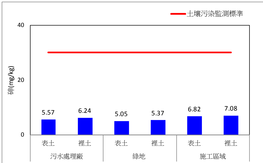
圖 2.4-7、109 年第二季土壤重金屬砷監測比較圖
