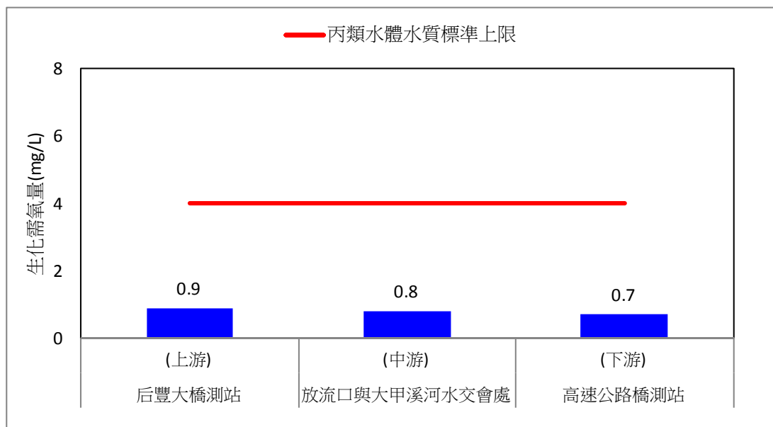
圖 2.1-2、109 年第二季地面水質生化需氧量監測比較圖
