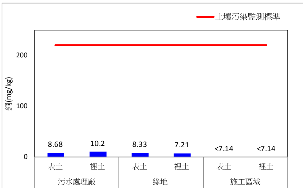
圖 2.4-2、109 年第二季土壤重金屬銅監測比較圖
