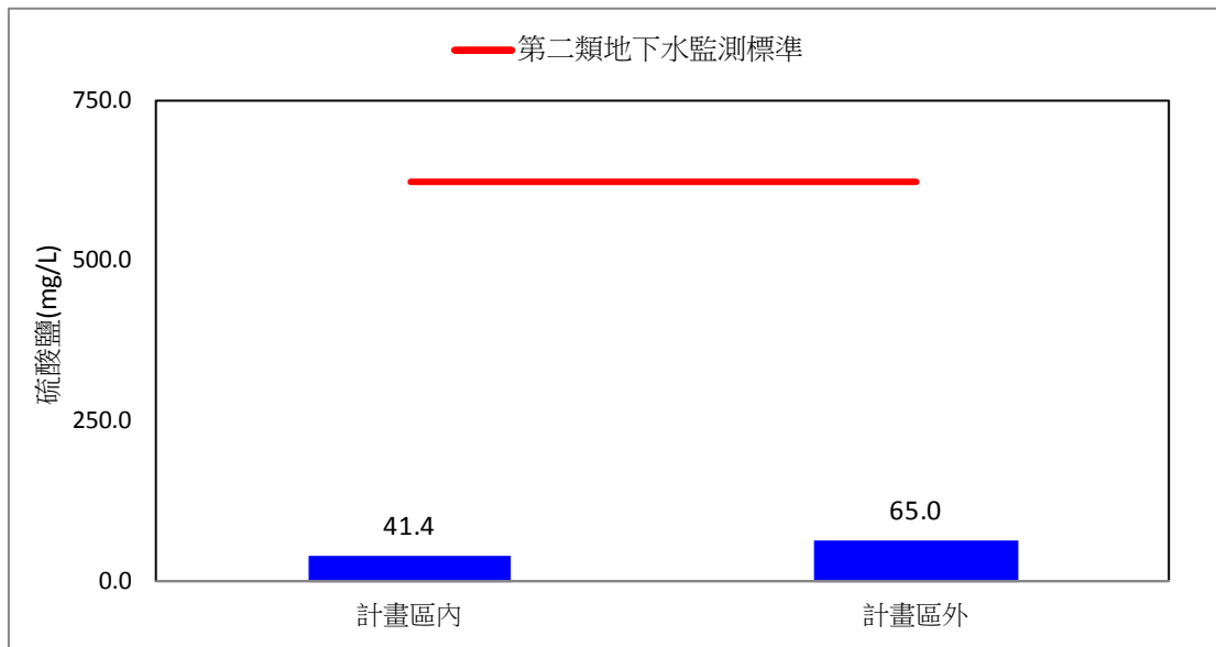
圖 2.2-1、109 年第二季地下水質硫酸鹽監測比較圖
