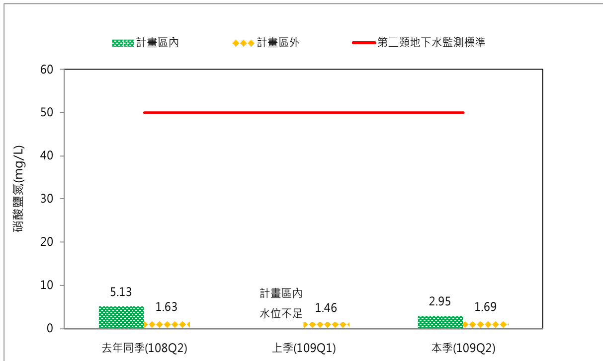
圖 3.1.1-22、本季、上季與去年同季施工暨營運期間地下水硝酸鹽氮監測成果
