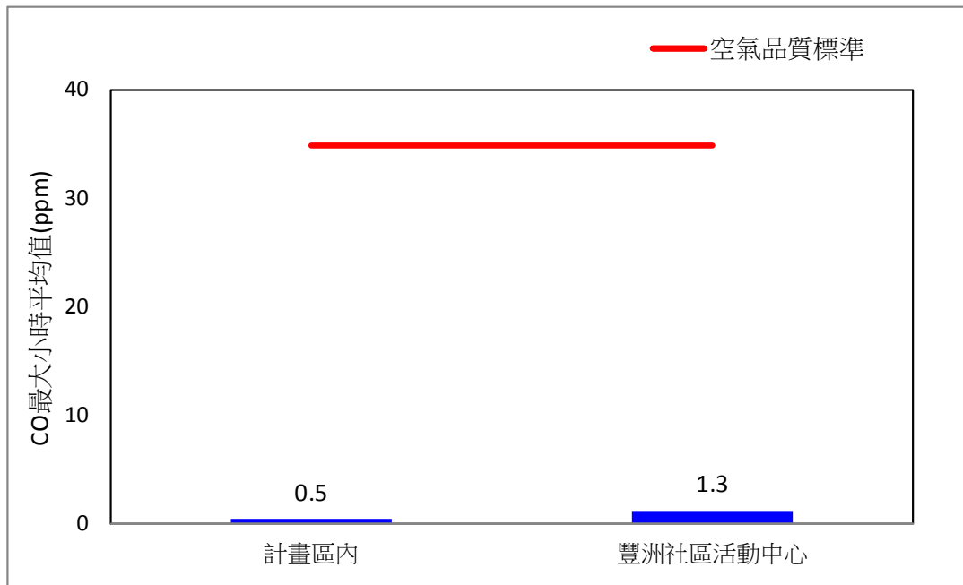
圖 2.3-5、109 年第二季空氣品質 CO 最大小時平均值監測比較圖
