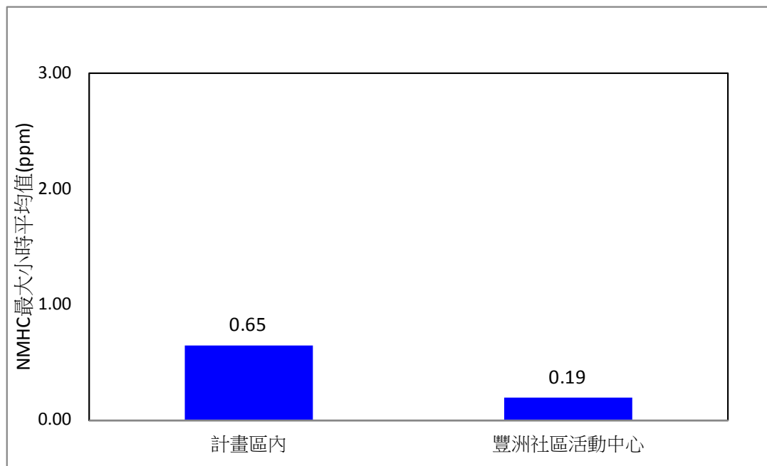
圖 2.3-12、109 年第二季空氣品質 NMHC 最大小時平均值監測比較圖
