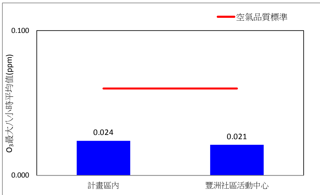
圖 2.3-10、109 年第二季空氣品質 O 3 最大八小時平均值監測比較圖
