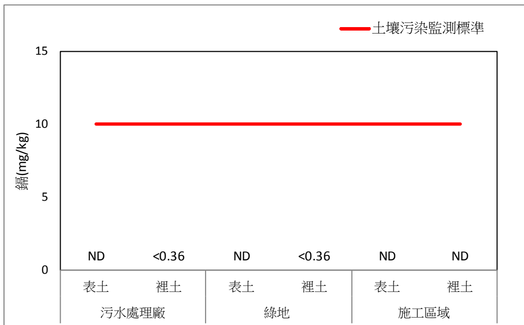
圖 2.4-4、109 年第二季土壤重金屬鎘監測比較圖
