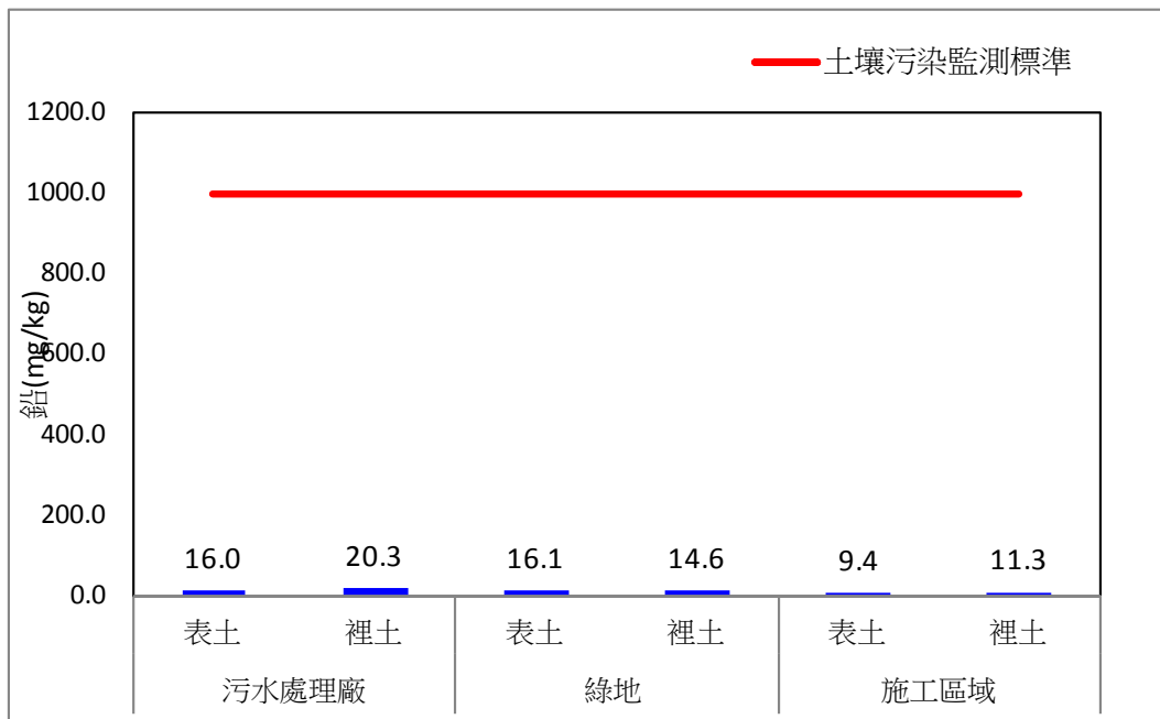
圖 2.4-1、109 年第二季土壤重金屬鉛監測比較圖
