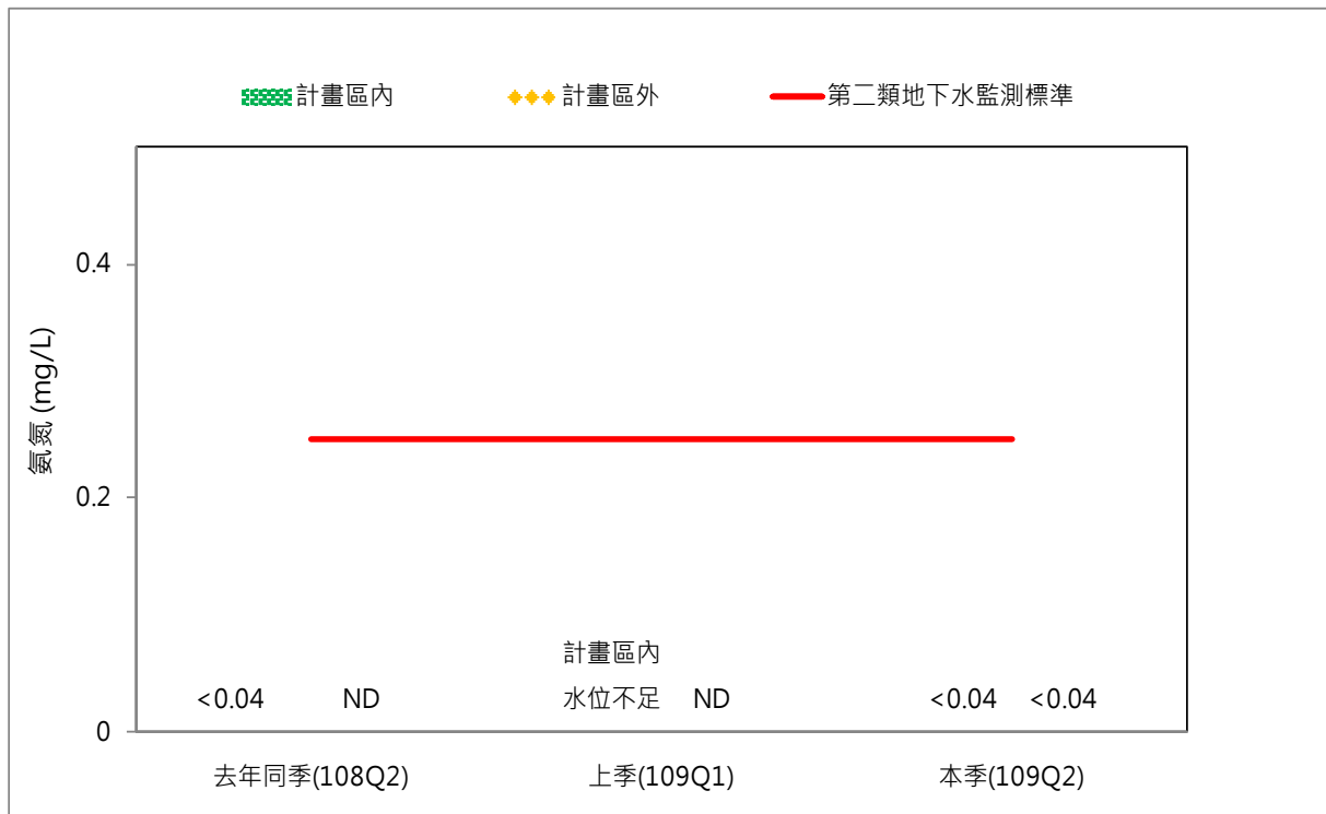
圖 3.1.1-24、本季、上季與去年同季施工暨營運期間地下水氨氮監測成果
