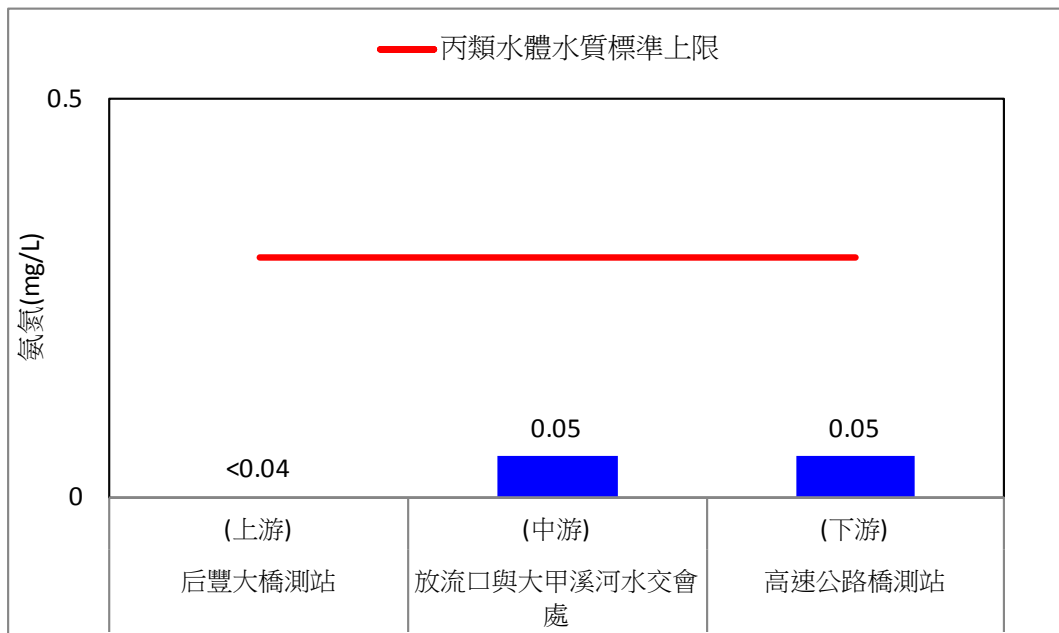
圖 2.1-5、109 年第二季地面水質氨氮監測比較圖
