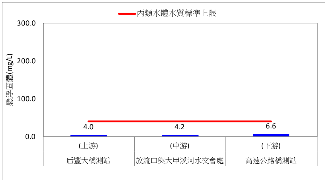
圖 2.1-3、109 年第二季地面水質懸浮固體監測比較圖
