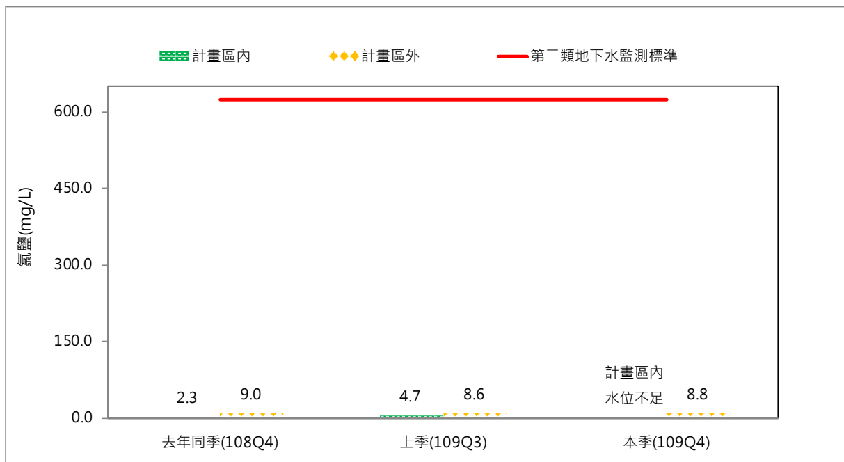
圖 3.1.1-23、本季、上季與去年同季施工暨營運期間地下水氟鹽監測成果
