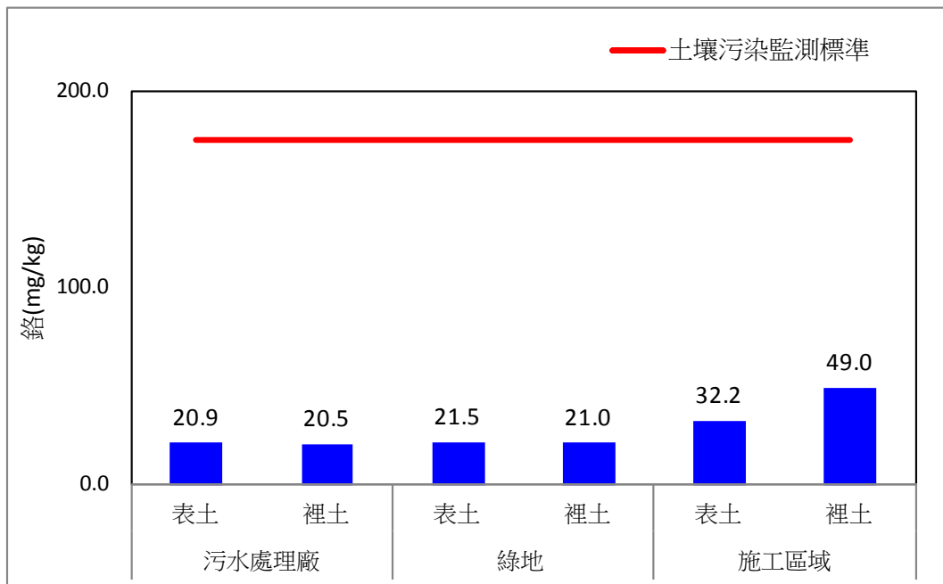
圖 2.4-5、109 年第四季土壤重金屬鉻監測比較圖
