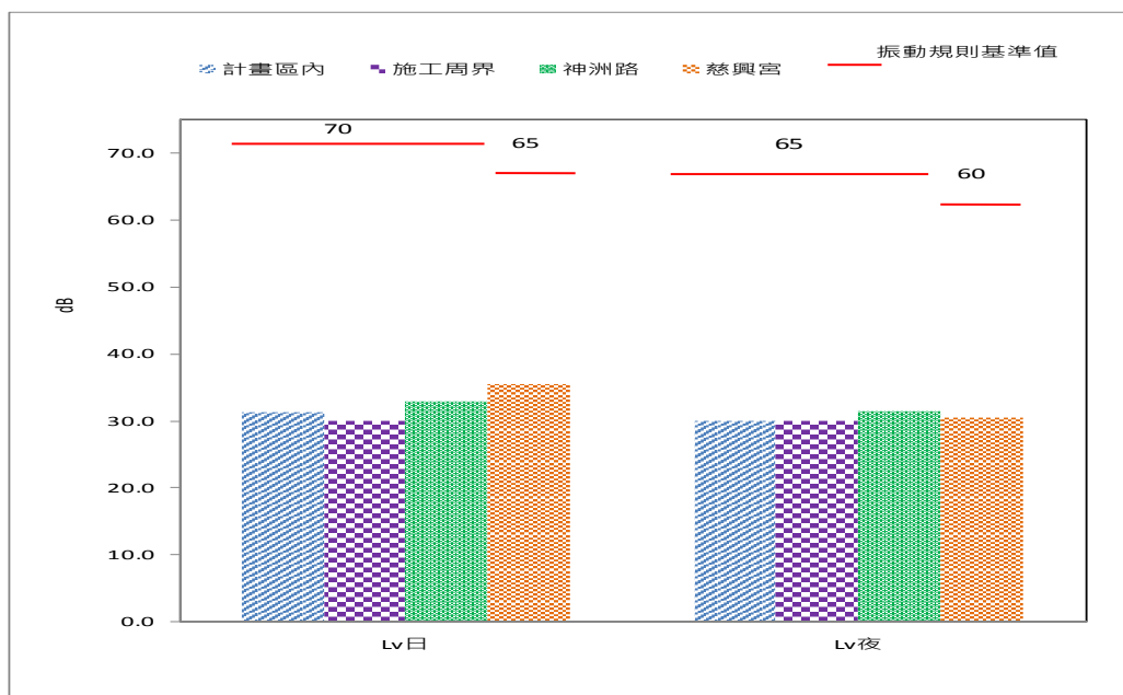
圖 2.5-2、109 年第四季各時段振動監測值比較圖
