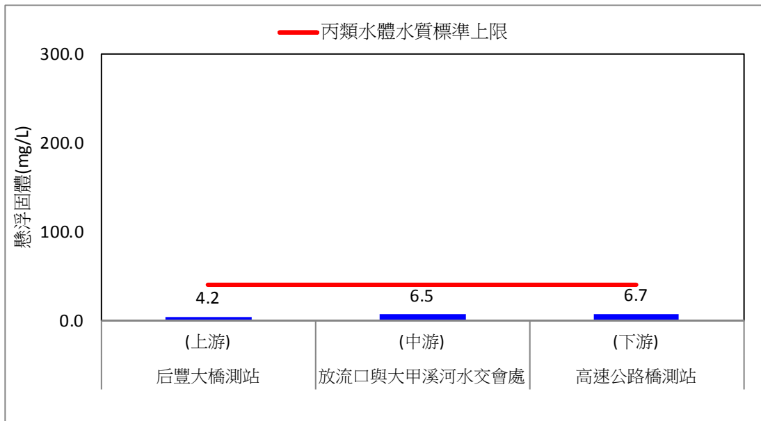
圖 2.1-3、109 年第四季地面水質懸浮固體監測比較圖
