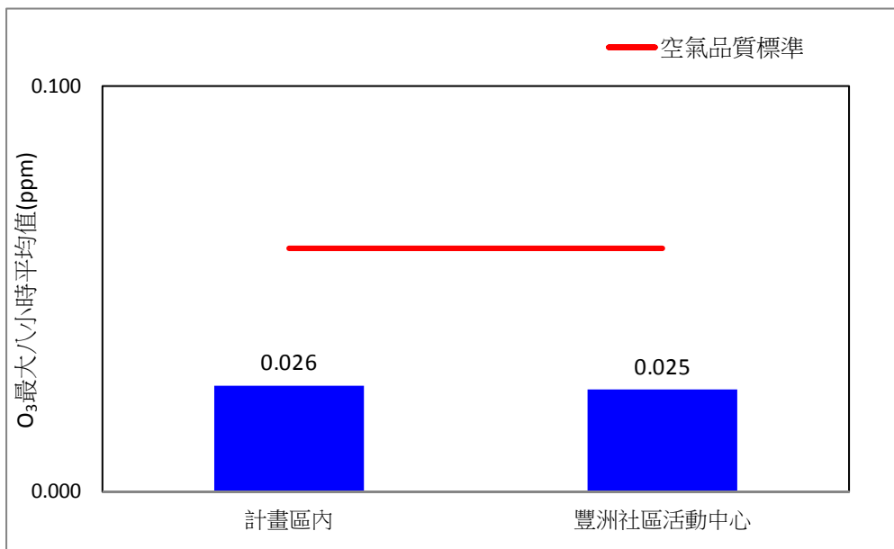
圖 2.3-10、109 年第四季空氣品質 O 3 最大八小時平均值監測比較圖
