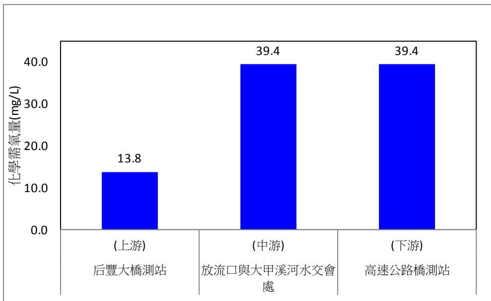
圖 2.1-8、109 年第四季地面水質化學需氧量監測比較圖
