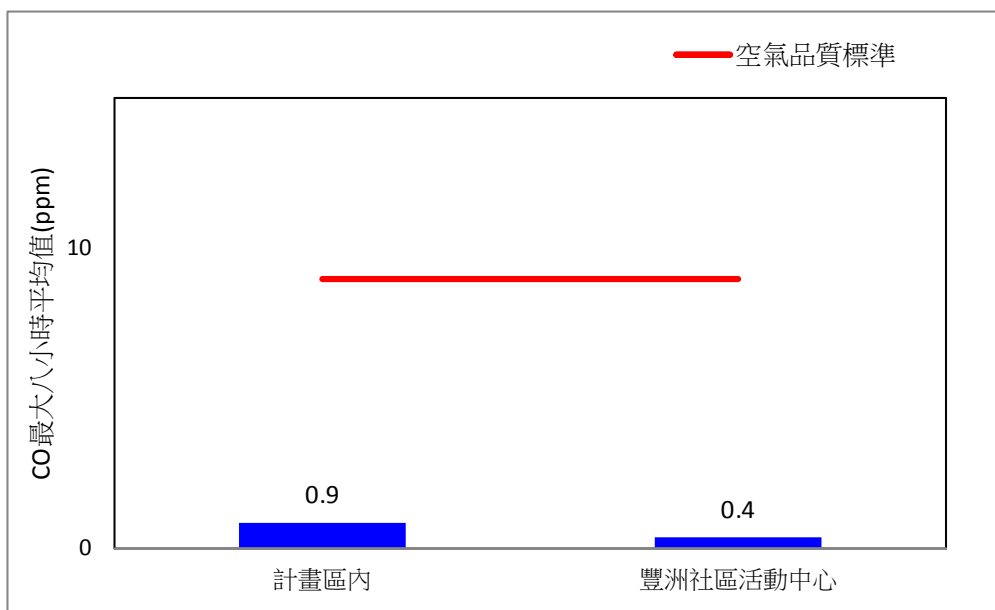
圖 2.3-6、109 年第四季空氣品質 CO 最大八小時平均值值監測比較圖
