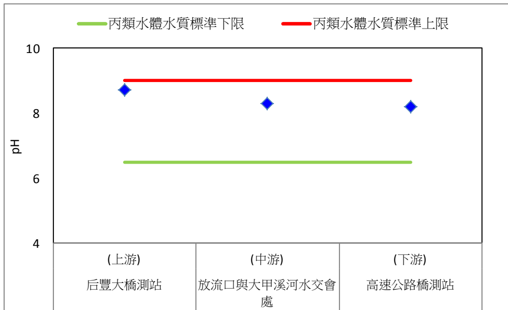
圖 2.1-1、109 年第四季地面水質 pH 值監測比較圖
