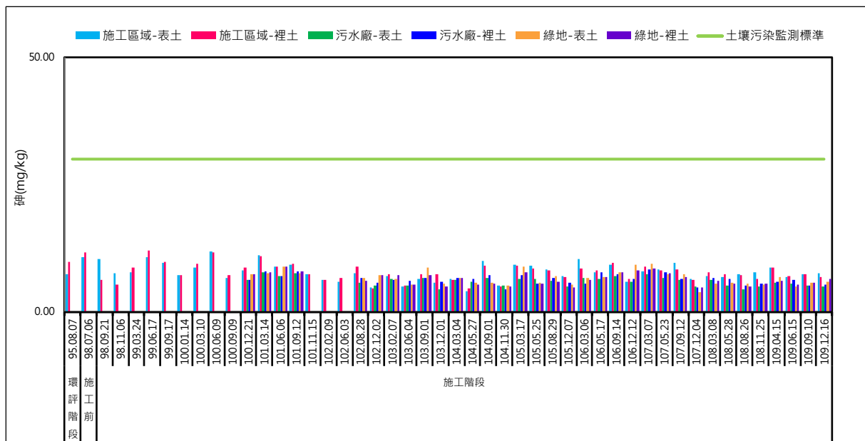
圖 3.1.1-65、歷次土壤重金屬砷監測結果
