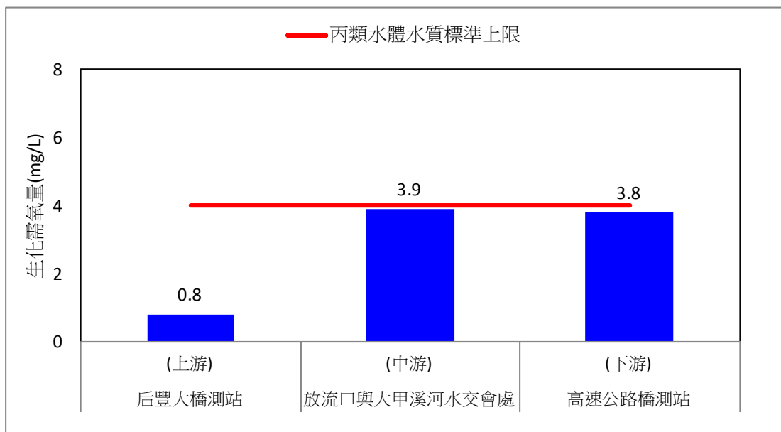
圖 2.1-2、109 年第四季地面水質生化需氧量監測比較圖
