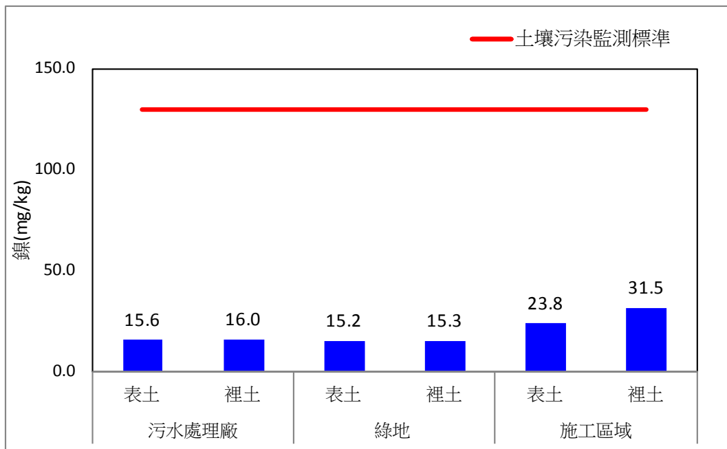
圖 2.4-6、109 年第四季土壤重金屬鎳監測比較圖
