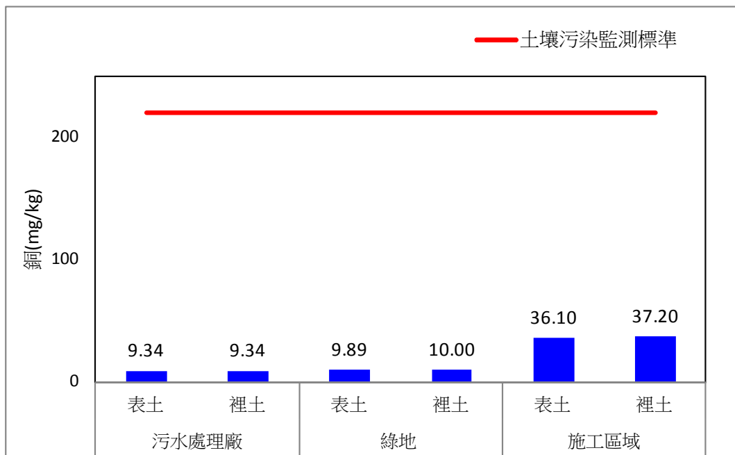
圖 2.4-2、109 年第四季土壤重金屬銅監測比較圖
