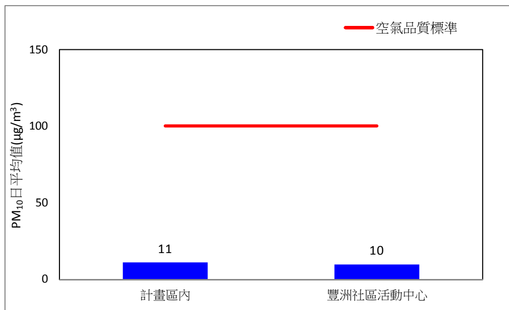
圖 2.3-2、109 年第四季空氣品質 PM 10 日平均值監測比較圖
