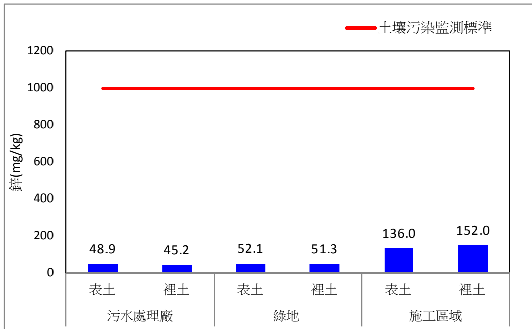
圖 2.4-3、109 年第四季土壤重金屬鋅監測比較圖
