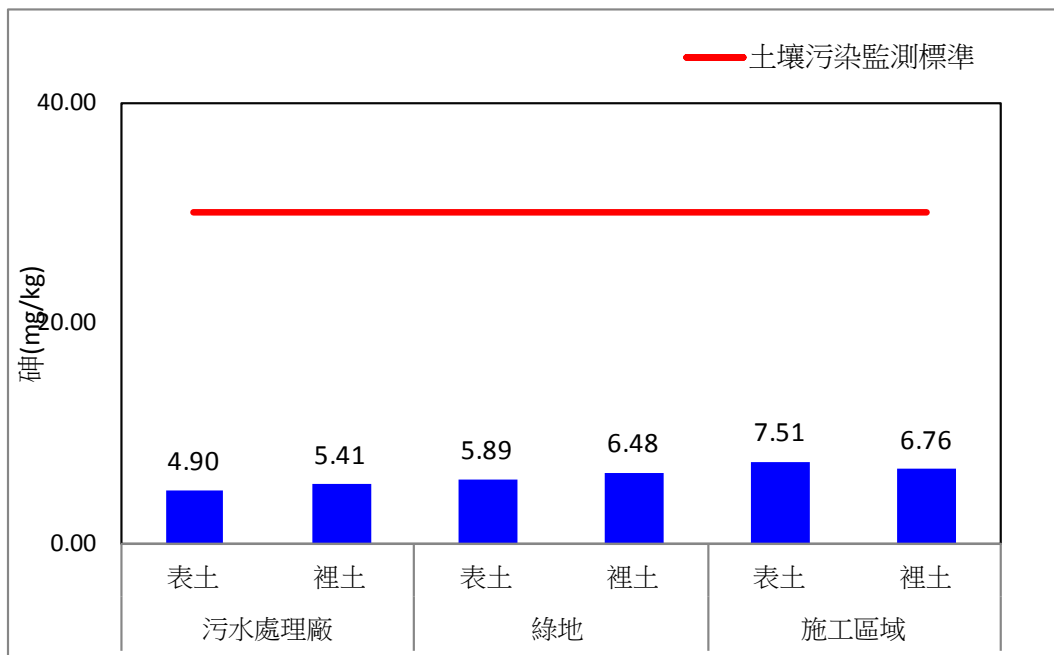
圖 2.4-7、109 年第四季土壤重金屬砷監測比較圖
