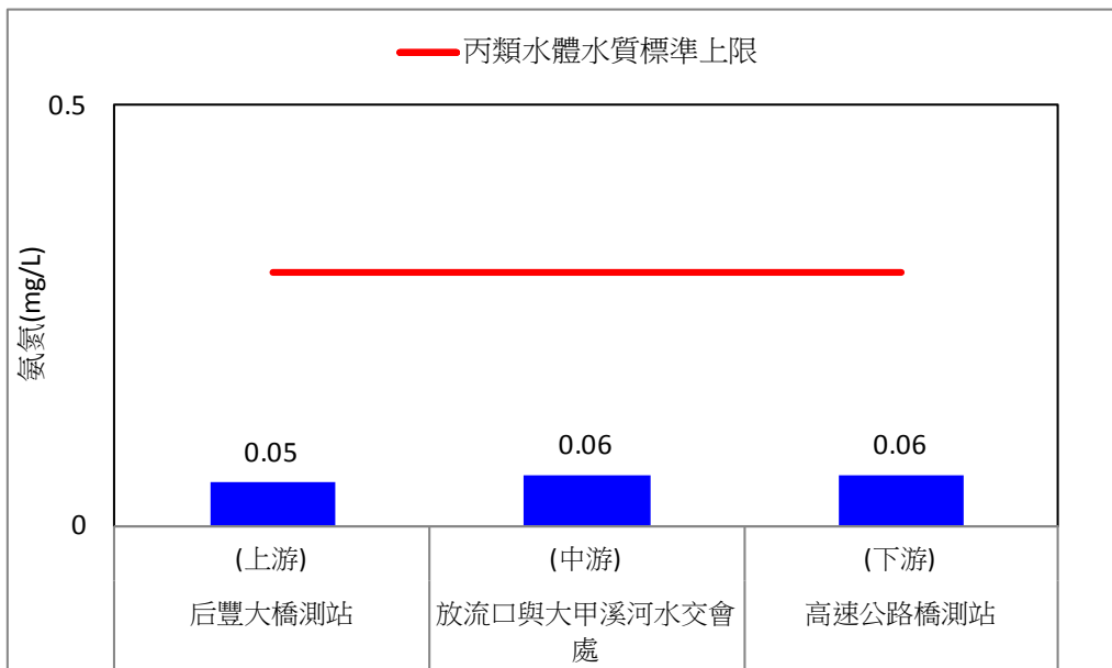
圖 2.1-5、109 年第四季地面水質氨氮監測比較圖
