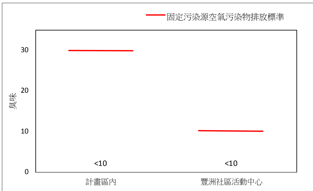
圖 2.3-14、109 年第四季空氣品質臭味監測比較圖
