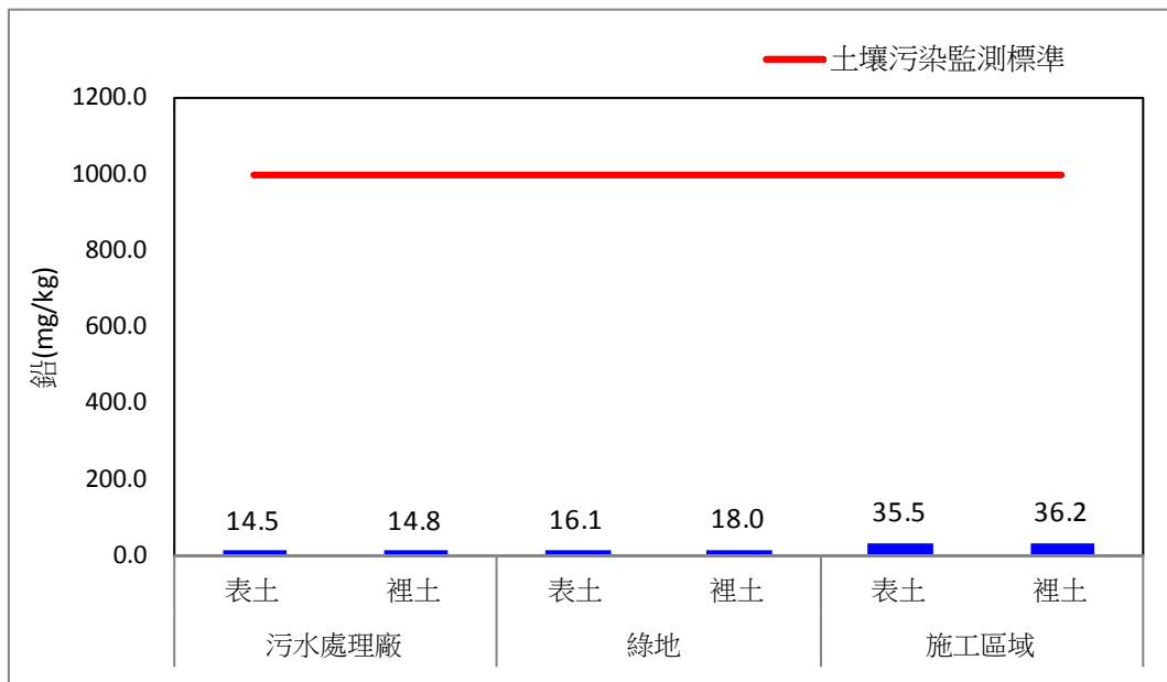
圖 2.4-1、109 年第四季土壤重金屬鉛監測比較圖
