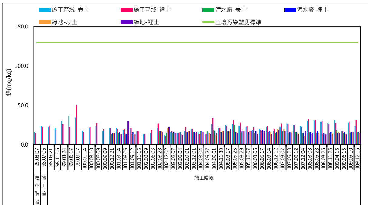
圖 3.1.1-64、歷次土壤重金屬鎳監測結果
