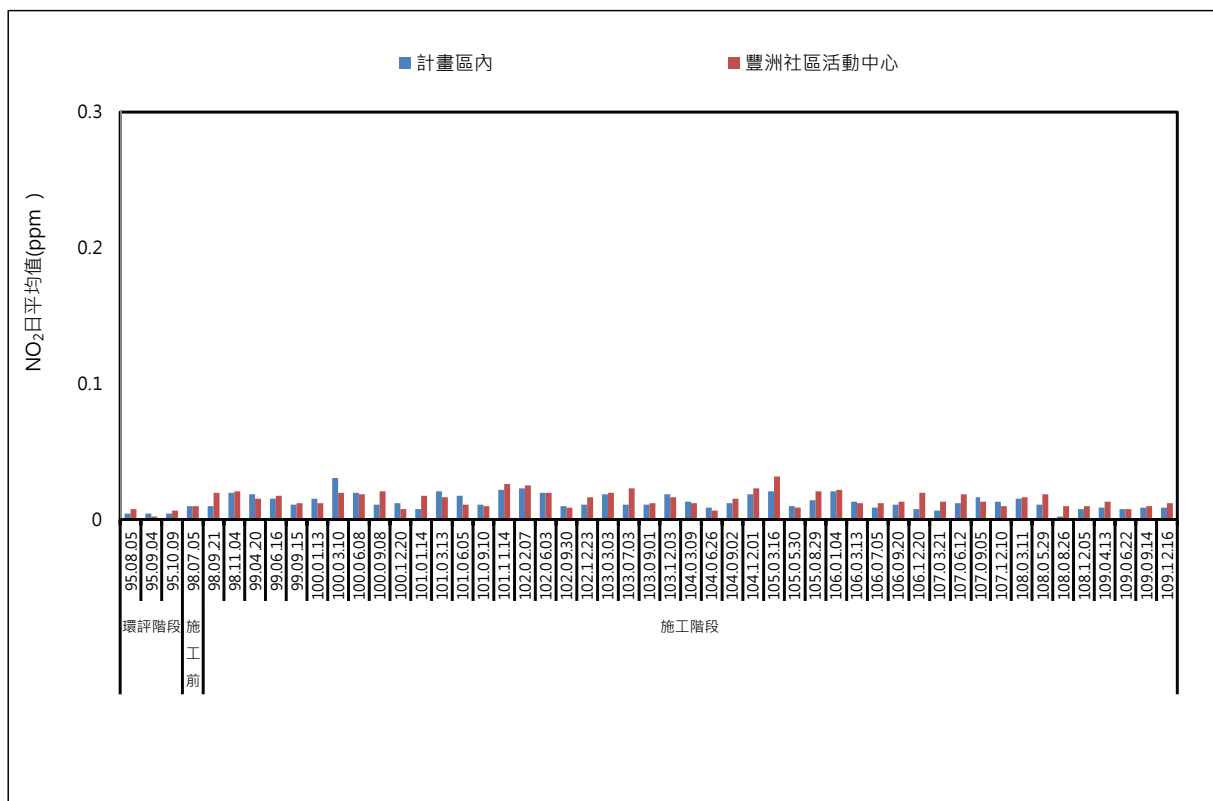
圖 3.1.1-49、歷次空氣品質 NO 2 日平均值監測結果
