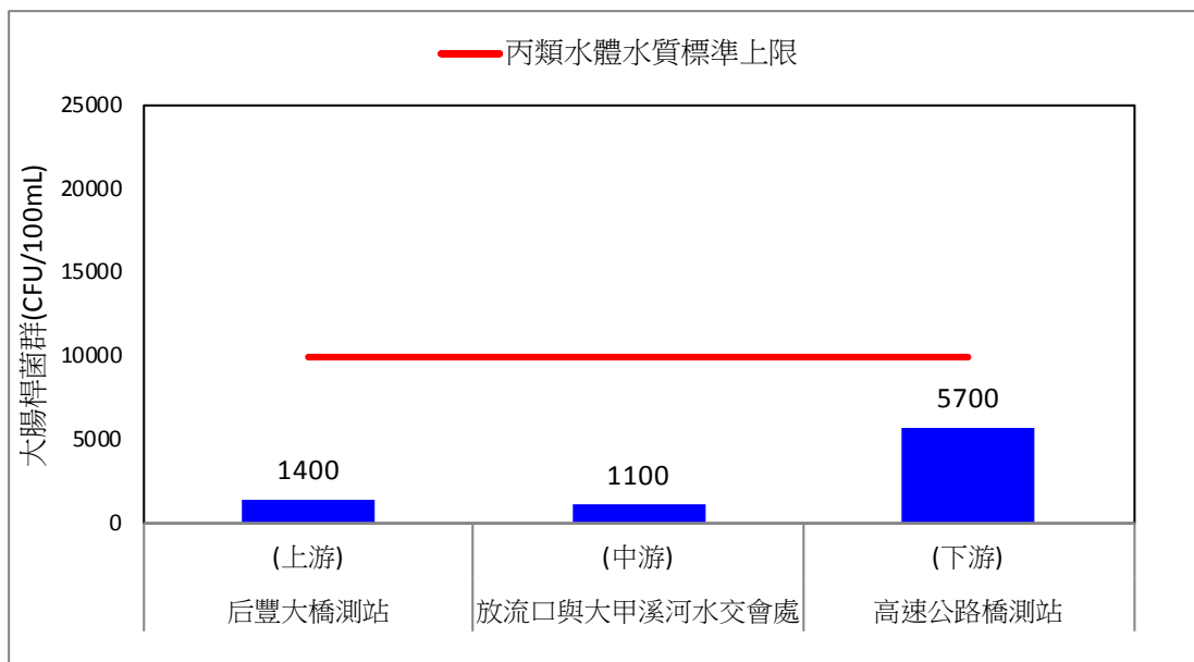
圖 2.1-4、109 年第四季地面水質大腸桿菌群監測比較圖
