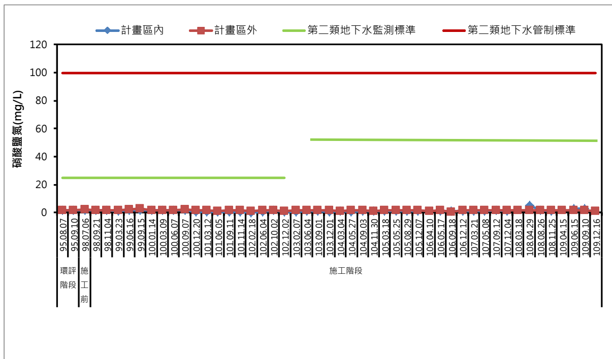
圖 3.1.1-30、歷次地下水質硝酸鹽氮監測結果
