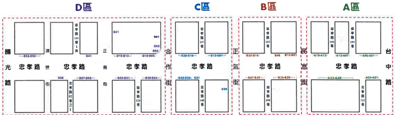
圖 1 忠孝路觀光夜市攤販集中區攤位配置圖(全區)
