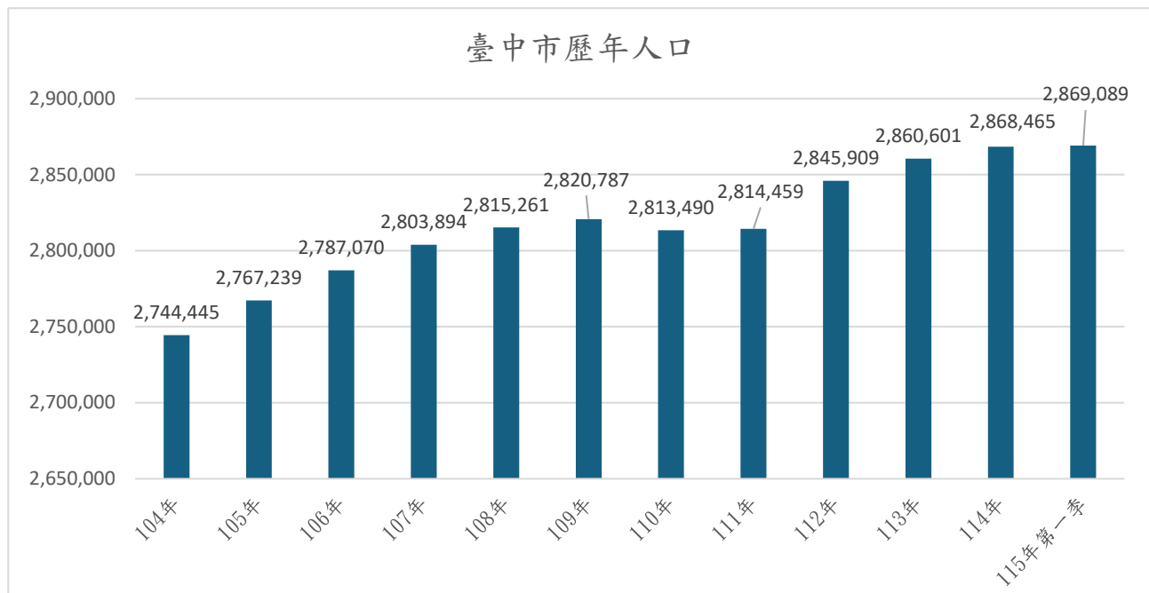
圖 2 臺中市歷年人口成長趨勢
