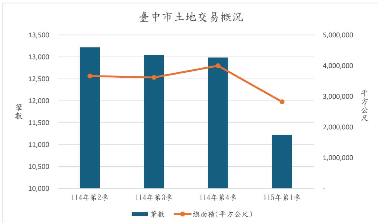
圖 13 臺中市土地交易概況
