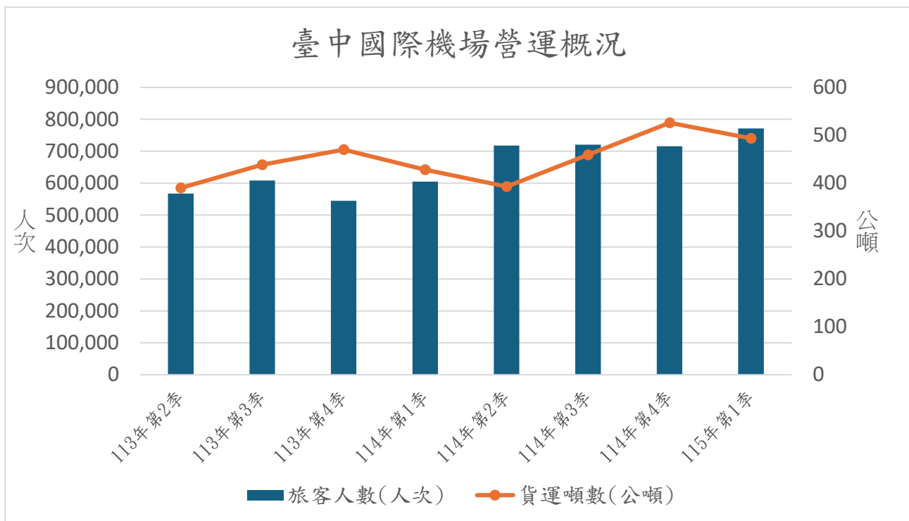
圖 21 臺中國際機場營運概況
