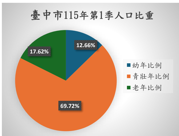
圖 1 臺中市 115 年第 1 季人口比重
