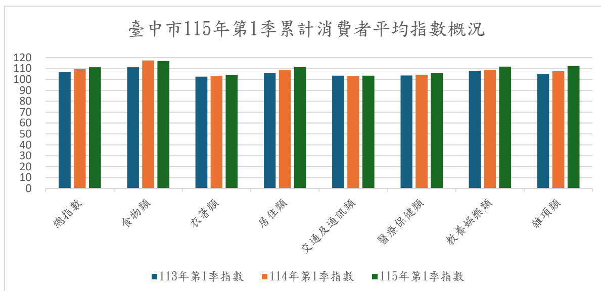
圖 5 臺中市 115 年第 1 季累計消費者平均指數概況
