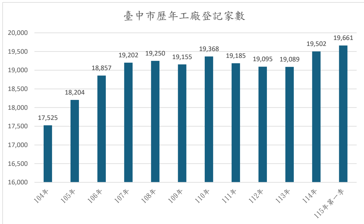
圖 10 臺中市歷年工廠登記家數成長趨勢
