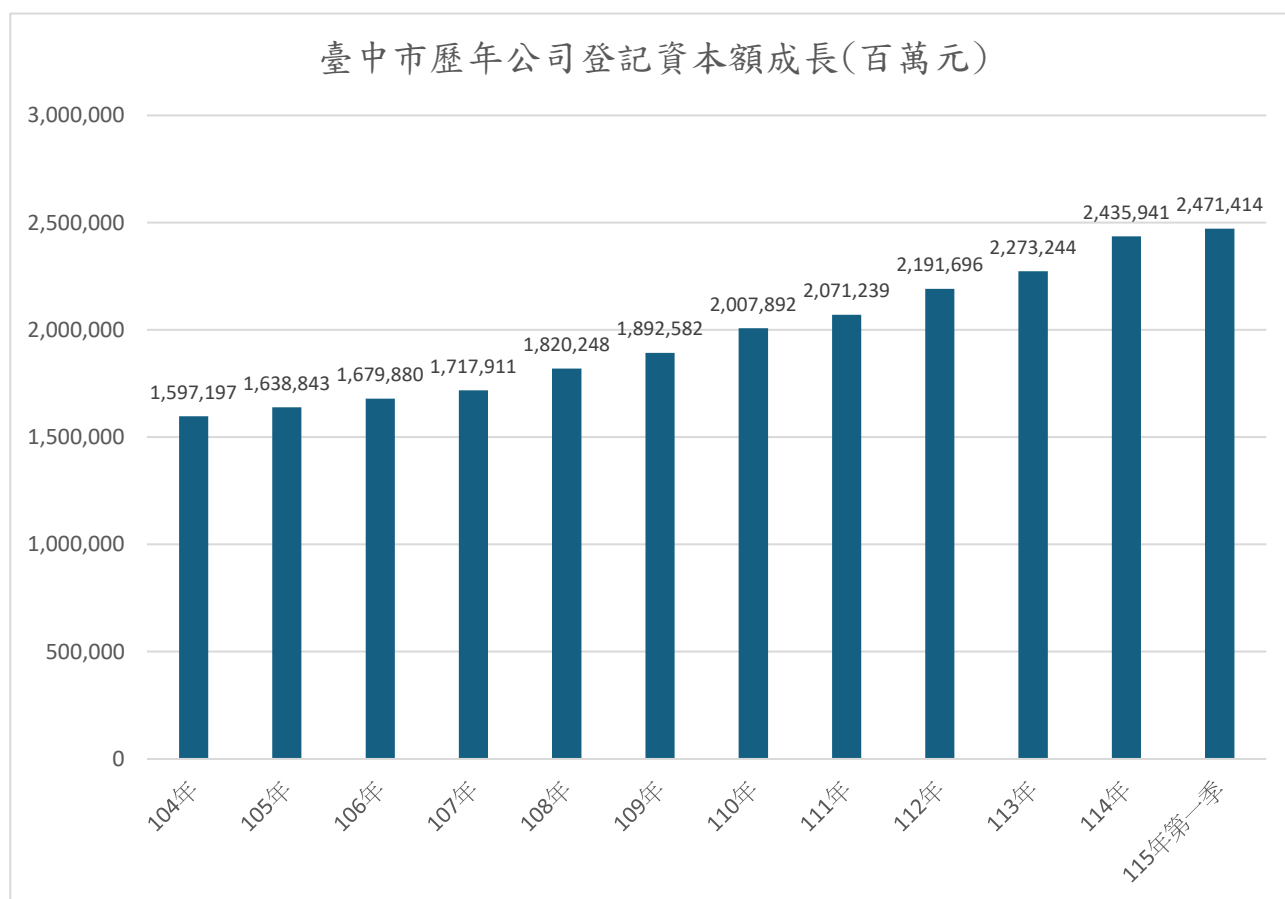
圖 7 臺中市歷年公司登記資本額成長趨勢
