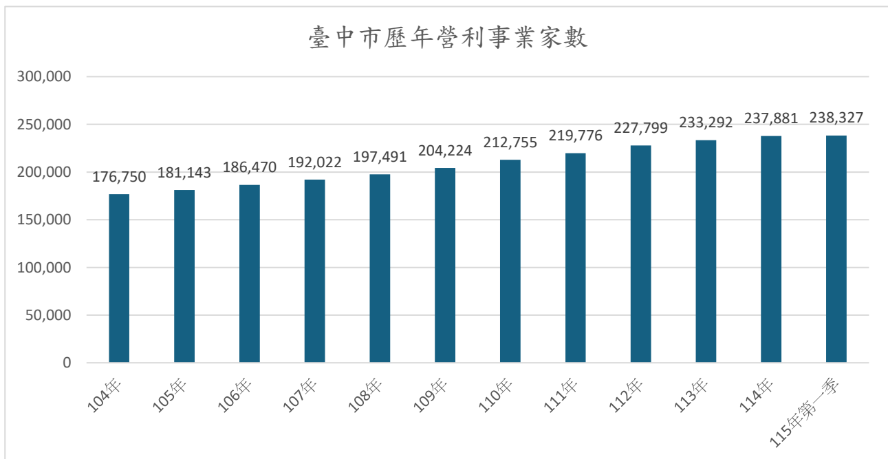
圖 3 臺中市歷年營利事業家數成長趨勢
