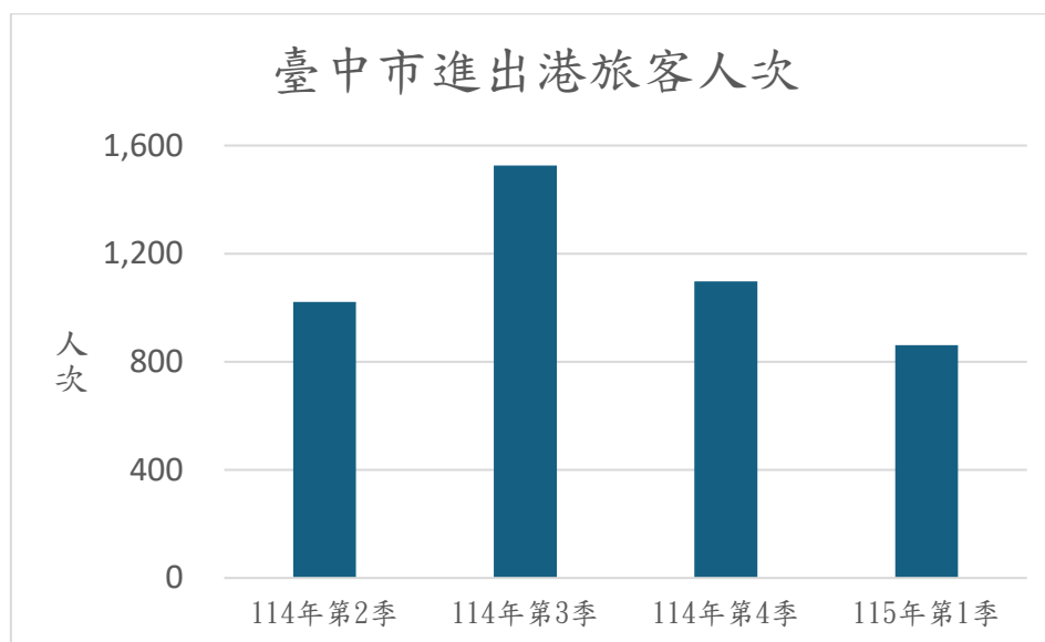
圖 18 臺中港最近四個季度進出港旅客人次概況
