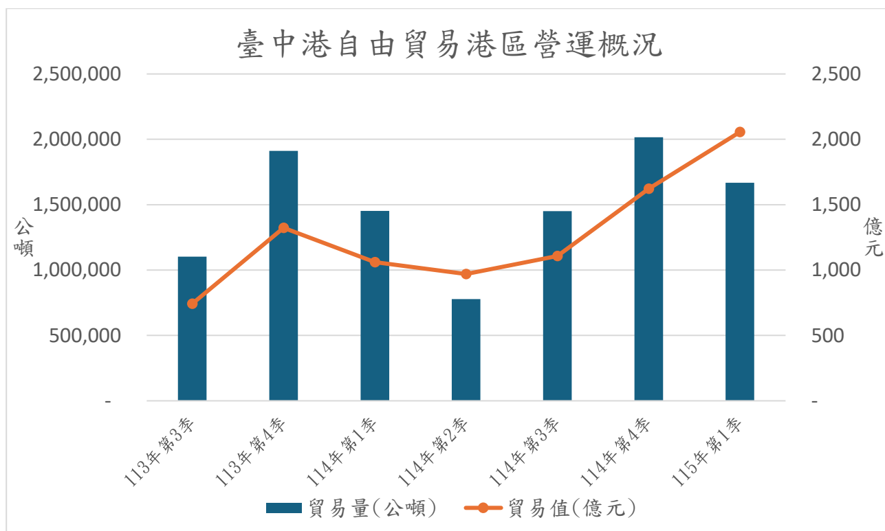
圖 20 臺中港自由貿易港區營運概況
