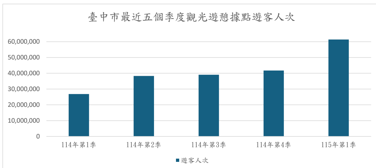
圖 16 臺中市最近五個季度觀光遊憩據點遊客人次
