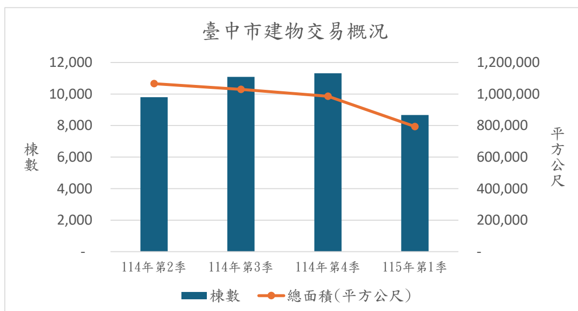
圖 14 臺中市建物交易概況
