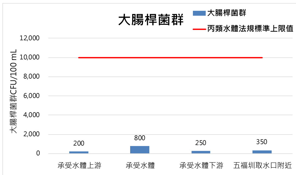
圖 2.5-6 本季地面水質大腸桿菌群監測結果分析圖
