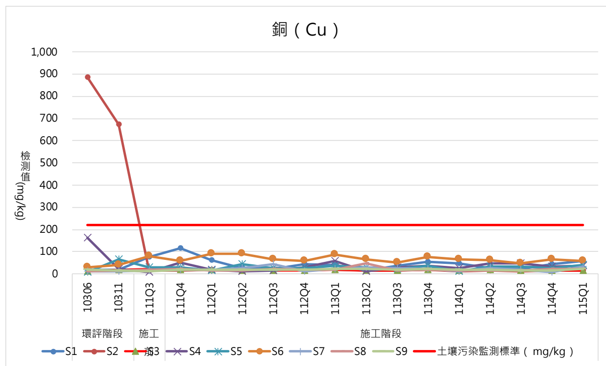
圖 2.7-15 歷年基地內土壤監測成果（銅）分析圖
