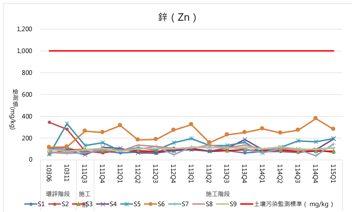
圖 2.7-19 歷年基地內土壤監測成果（鋅）分析圖
