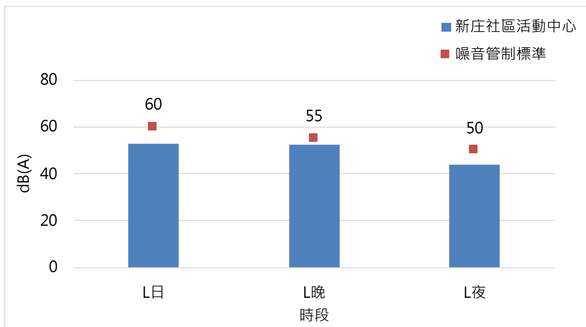
圖 2.1-1 本季新庄社區活動中心測站噪音監測成果分析圖
