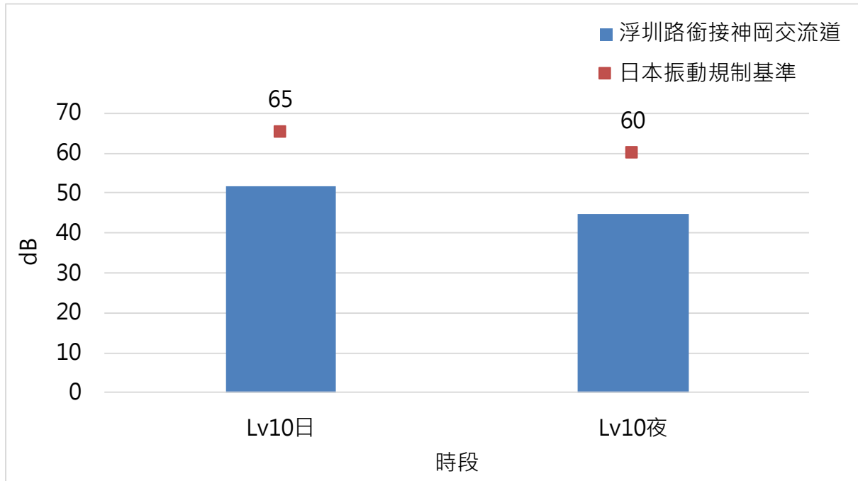
圖 2.1-10 本季浮圳路銜接神岡交流道測站振動監測成果分析圖
