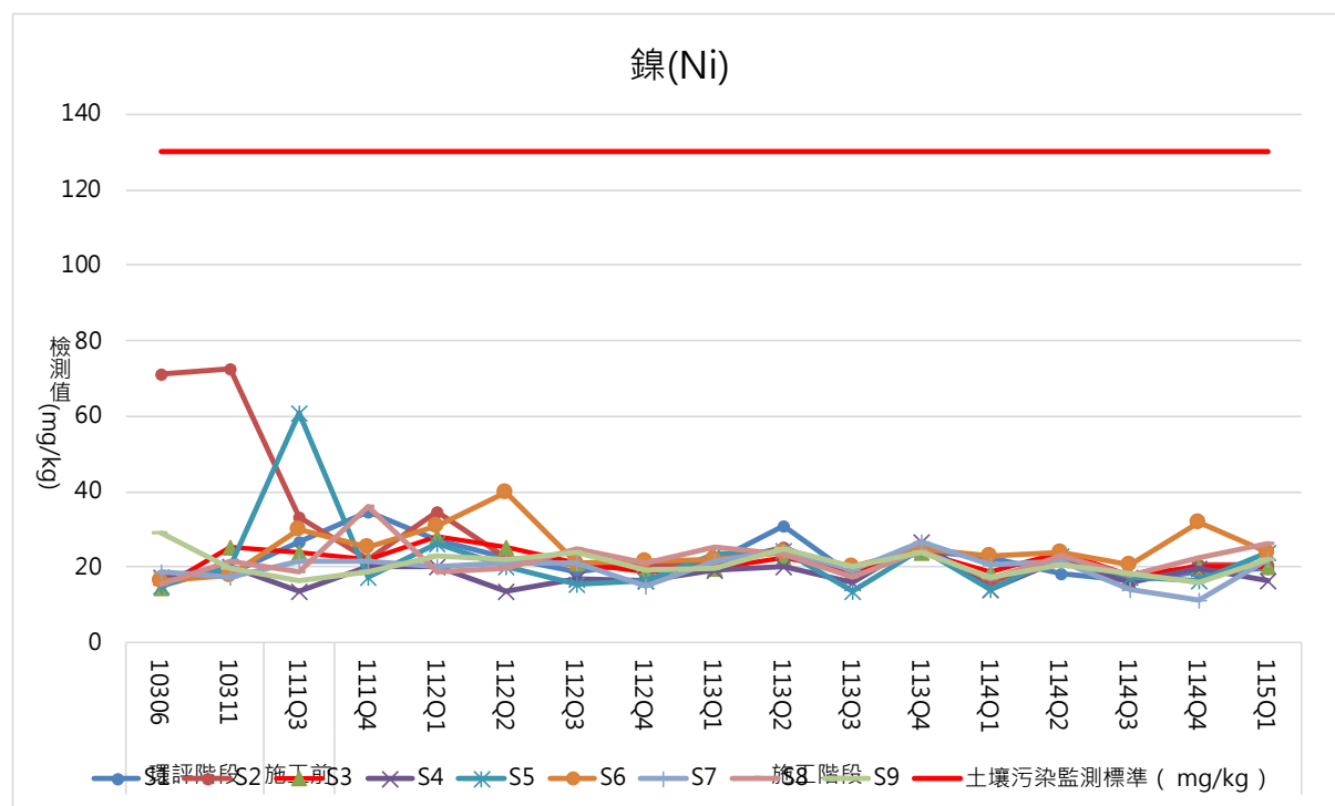
圖 2.7-17 歷年基地內土壤監測成果（鎳）分析圖
