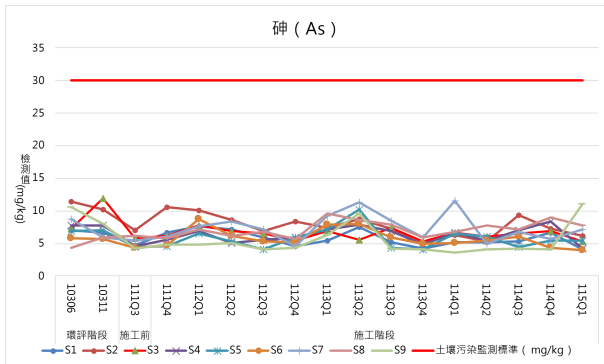
圖 2.7-12 歷年基地內土壤監測成果 (砷) 分析圖
