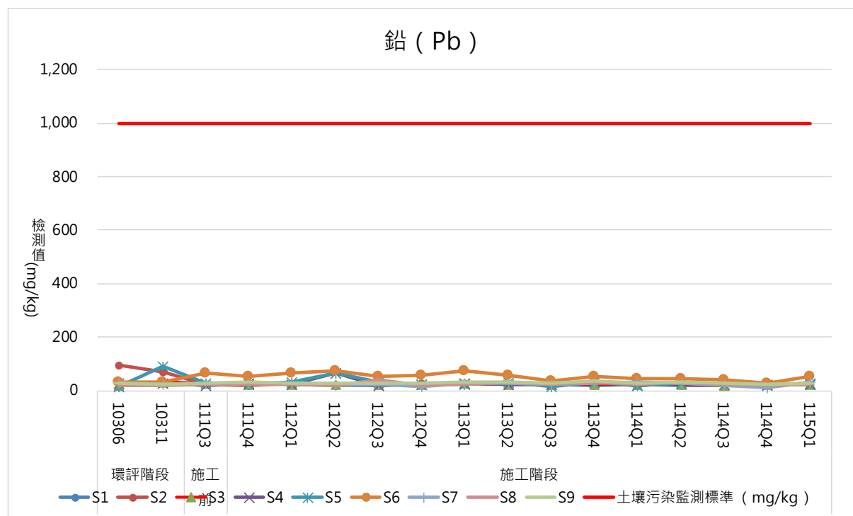
圖 2.7-18 歷年基地內土壤監測成果（鉛）分析圖
