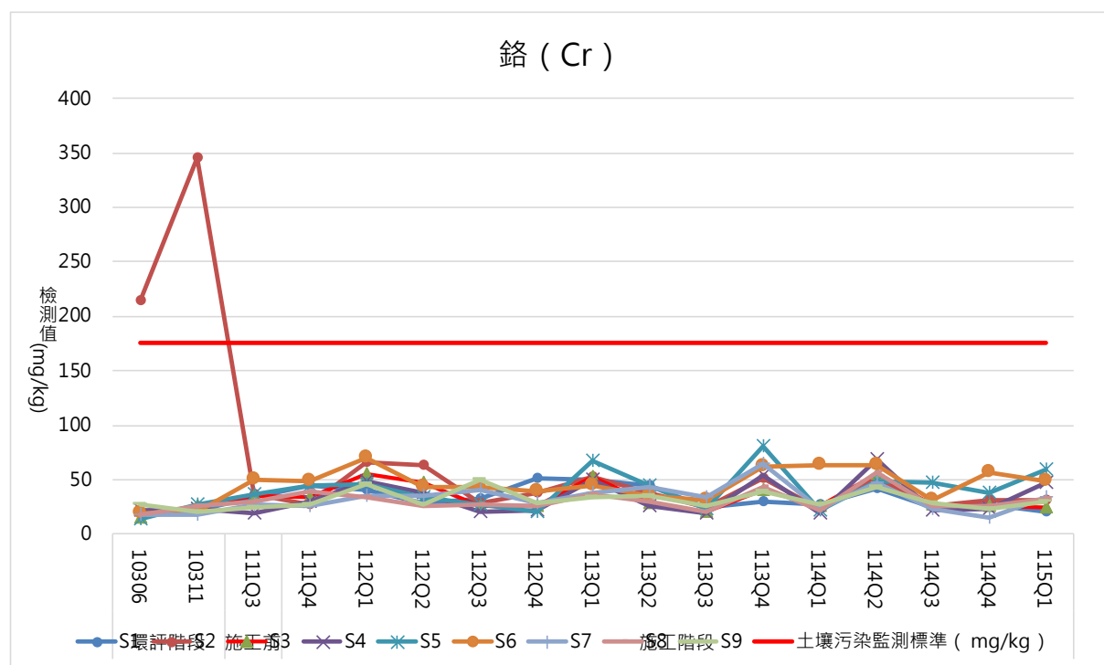
圖 2.7-14 歷年基地內土壤監測成果（鉻）分析圖
