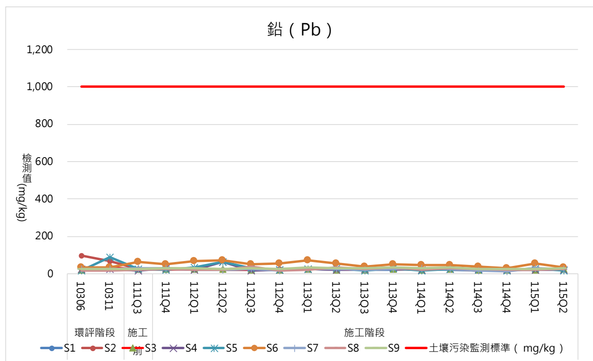
圖 2.7-18 歷年基地內土壤監測成果（鉛）分析圖
