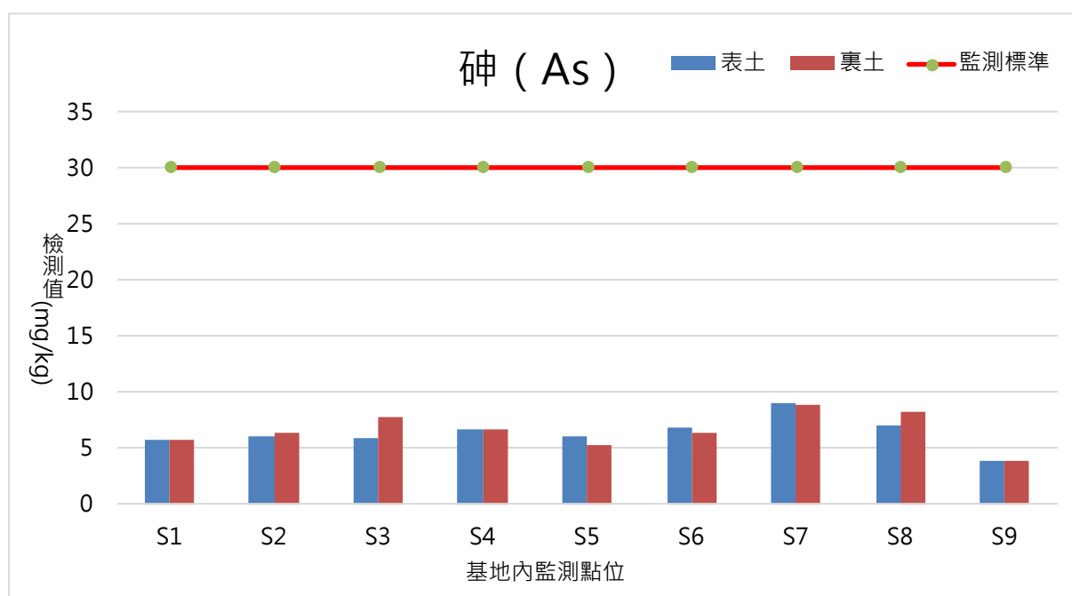
圖 2.7-3 本季基地內土壤監測成果 (砷) 分析圖
