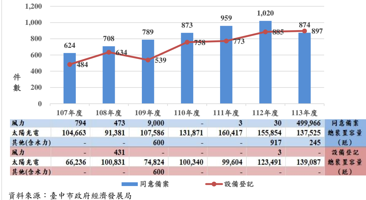
圖10 臺中市再生能源發電設備之核准情形
