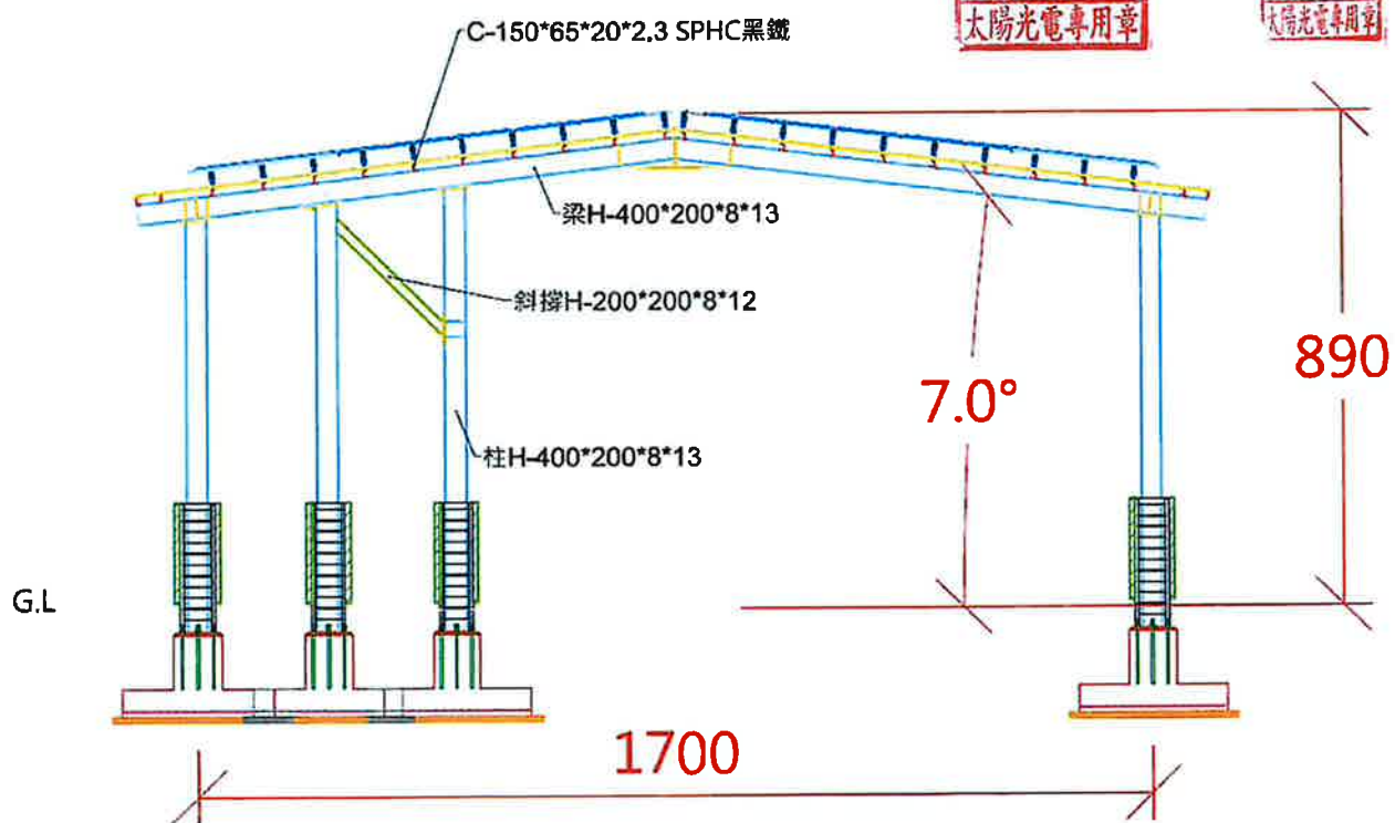
遊戲區東向立面圖
