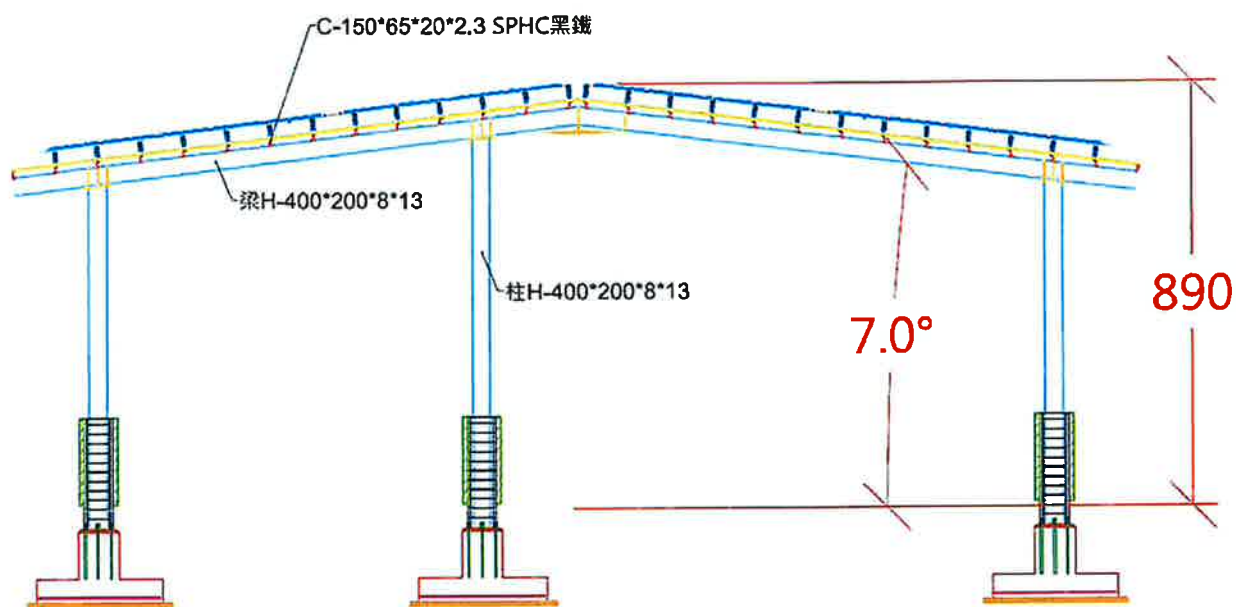
風雨球場東向立面圖
