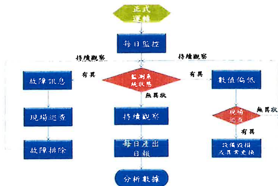
圖1-2 營運管理發電監控處理流程圖
