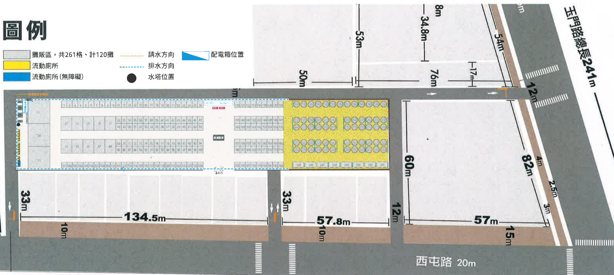
附圖三 攤位配置圖
